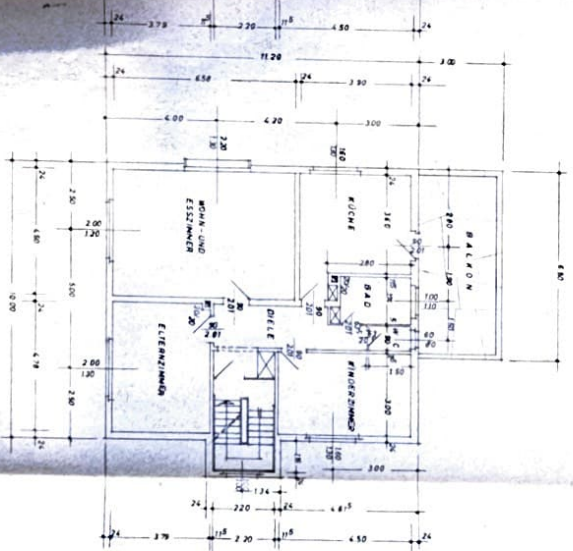
1. OBERGESCHOSS
