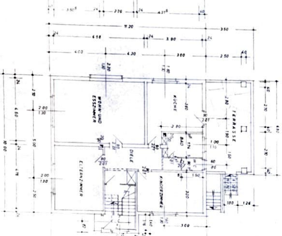
ERDGESCHOSS
