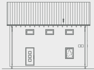
Ansicht Eingang
