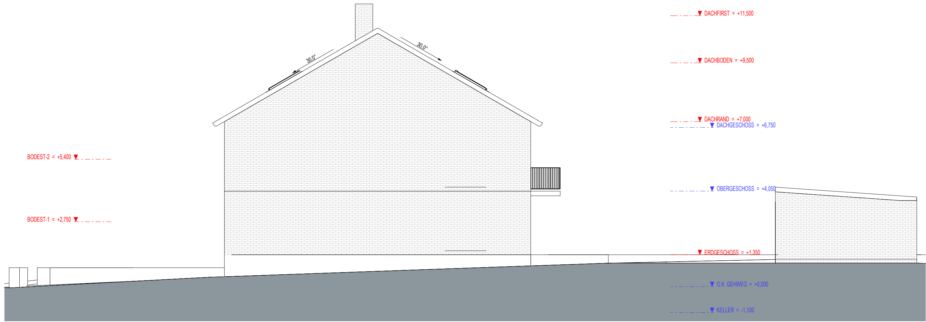
Ansicht 3 - Nord-West M 1 : 100
