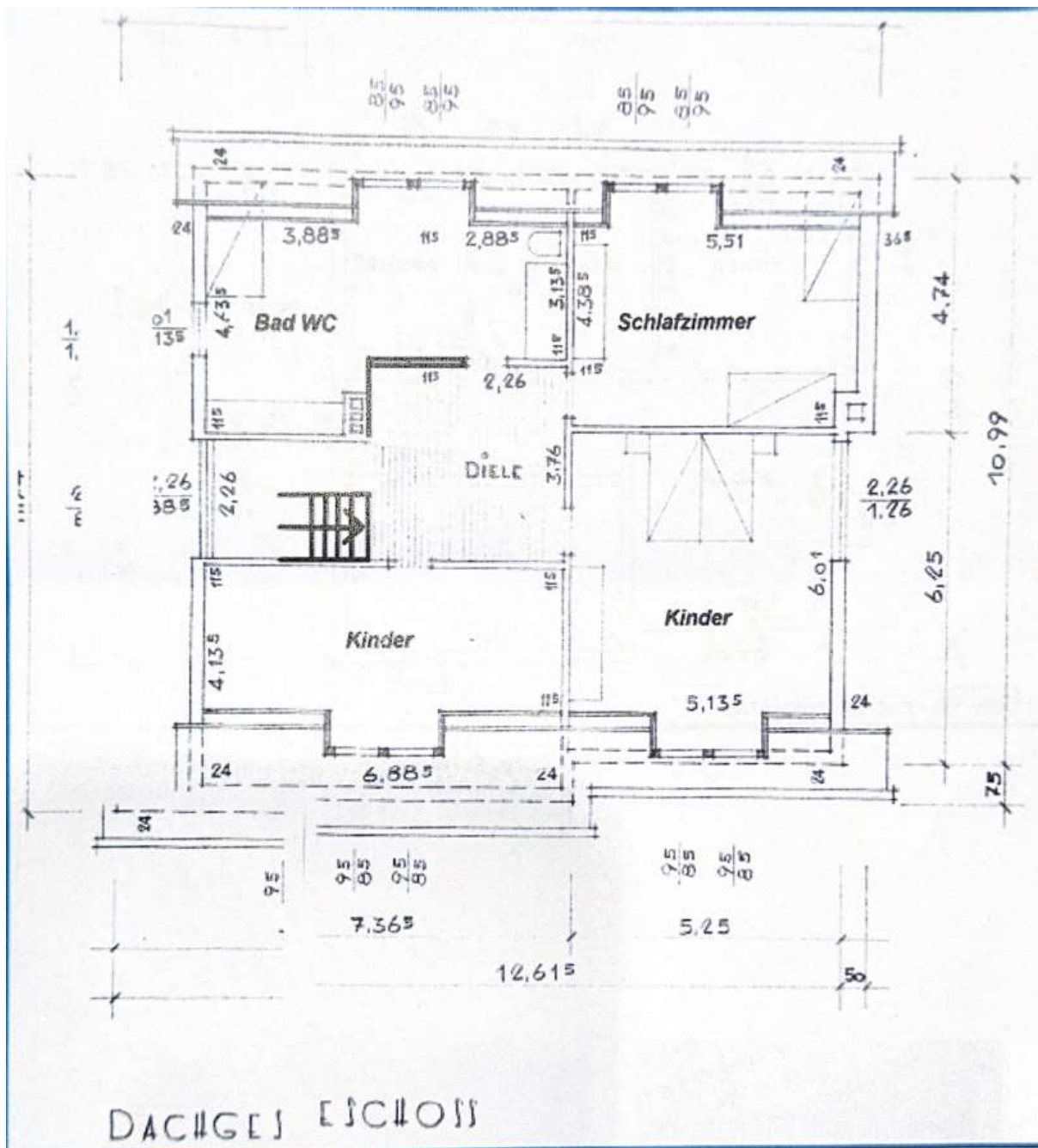
Obergeschoss
