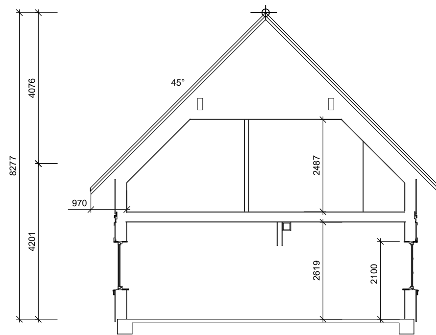
SCHNITT A-A
