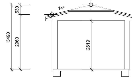
SCHNITT B-B
