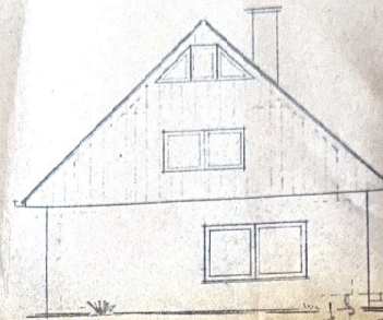
ANSICHT SÜD
