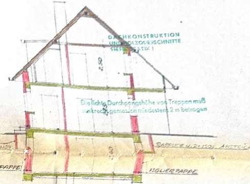
SCHNITT A-B
