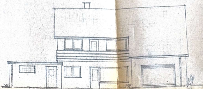
ANSICHT WEST
