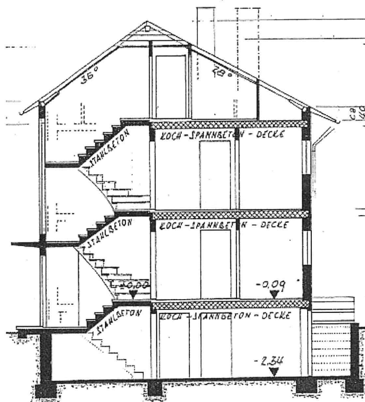
Schnitt
