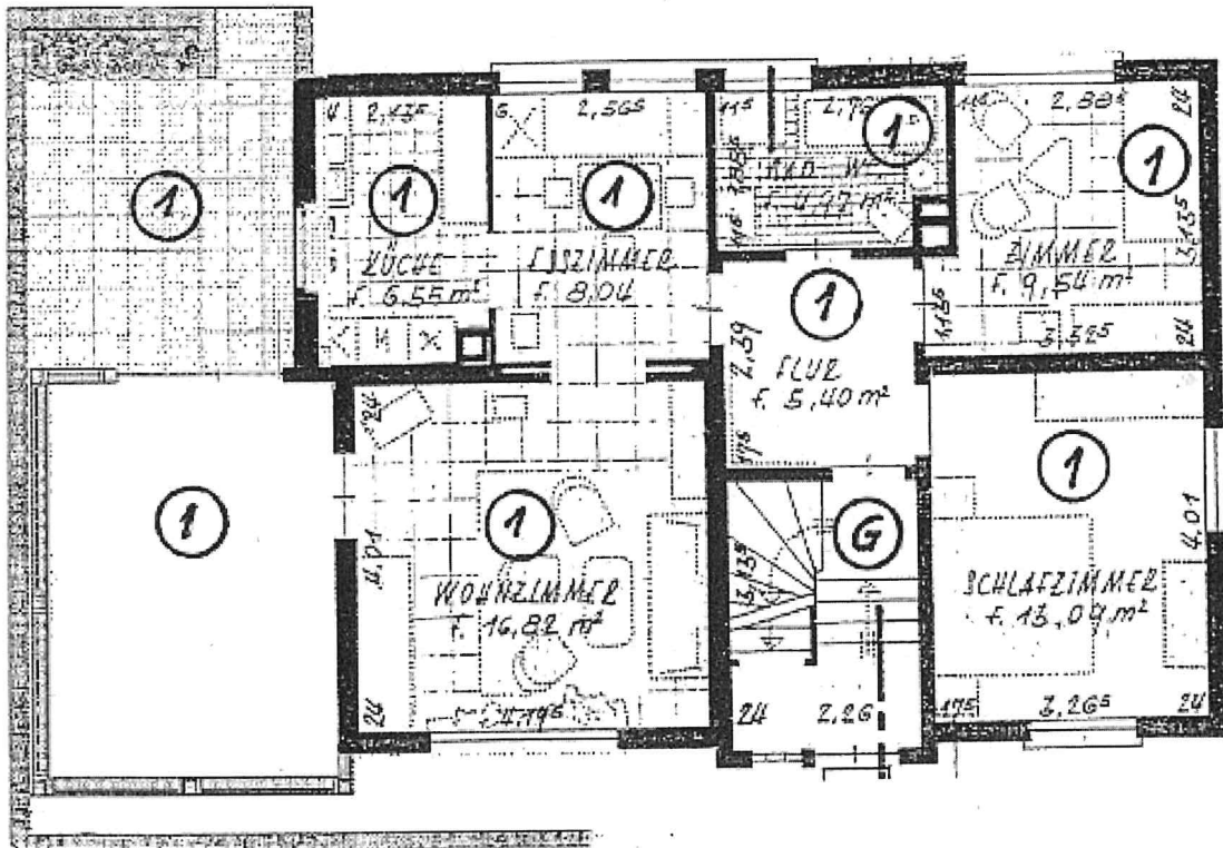
Erdgeschoss
