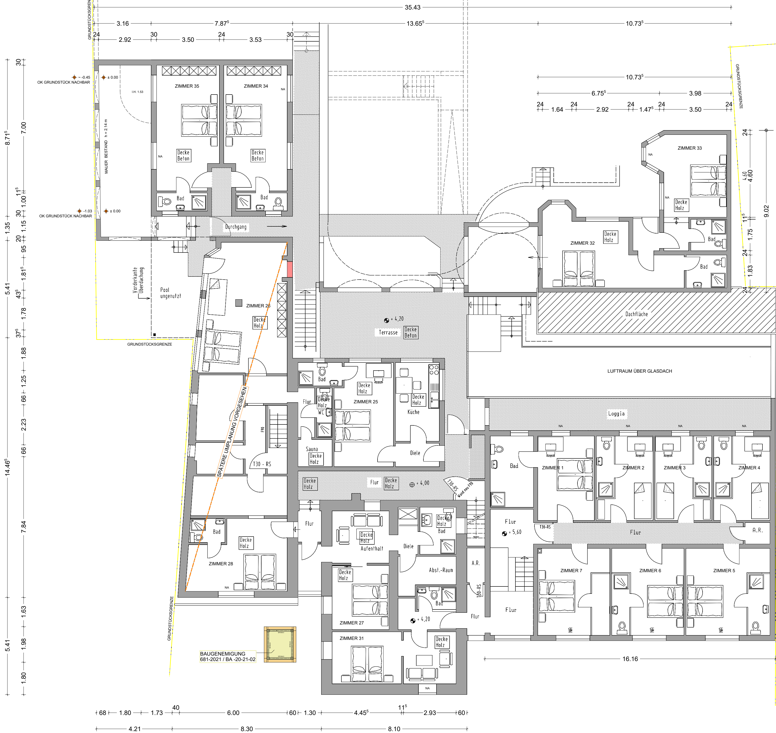
OBERGESCHOSS II
