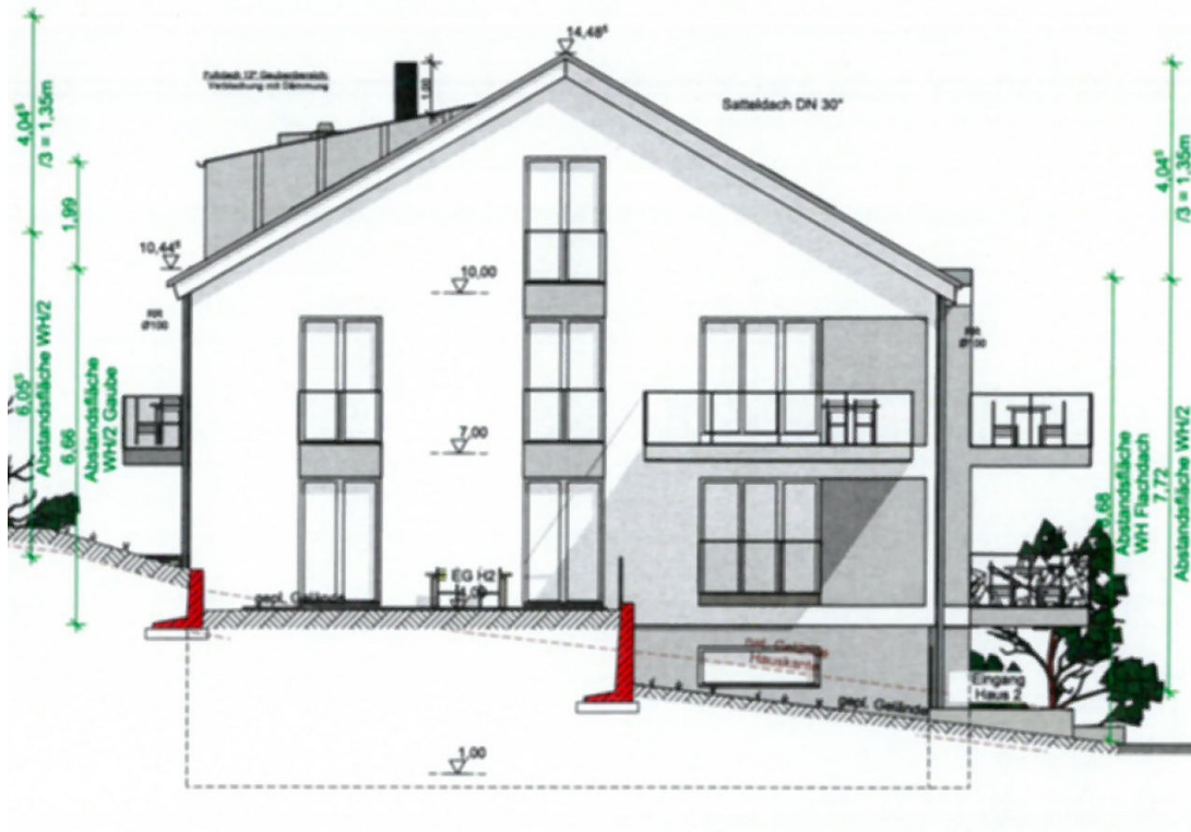
Nord H2 Ansicht Nord M 1:100
