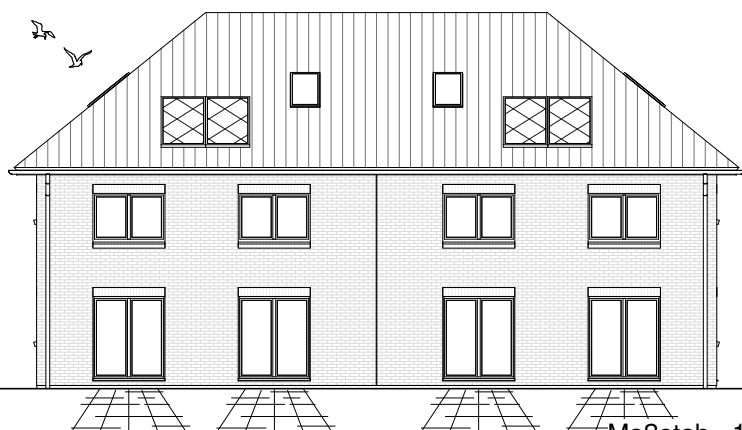
Maßstab 1 : 200
