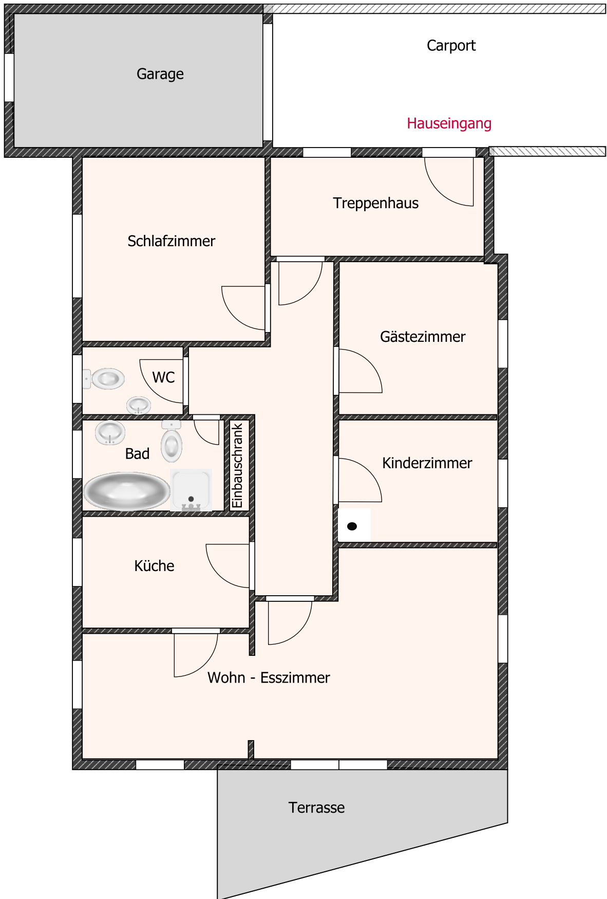
Grundriss Erdgeschoss nicht maßstabsgetreu
