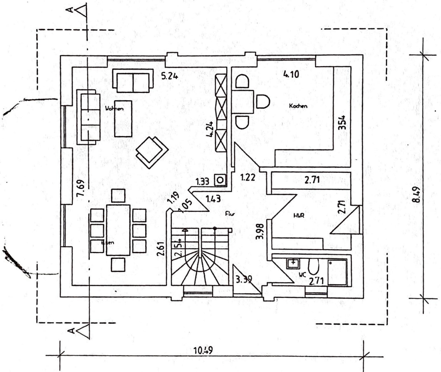
Erdgeschoss M. 1:100
