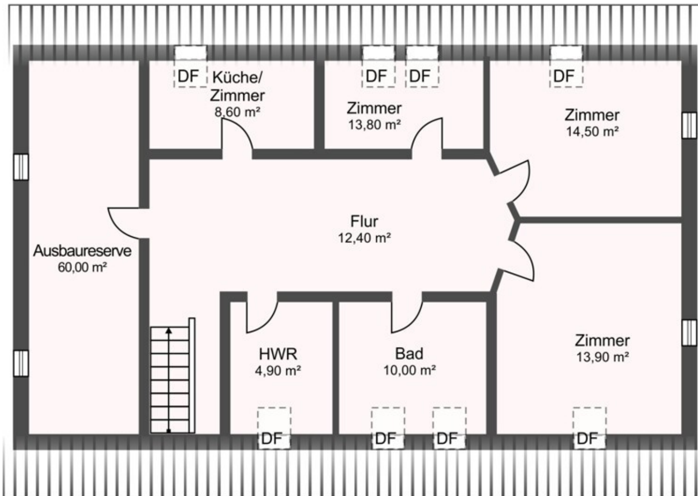
Dachgeschoss
