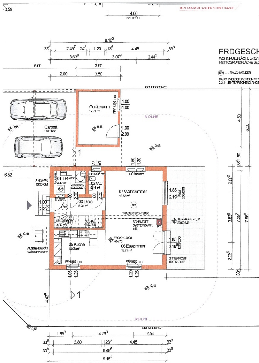
Neues 117m 2 Einfamilienwohnhaus in Viktring
