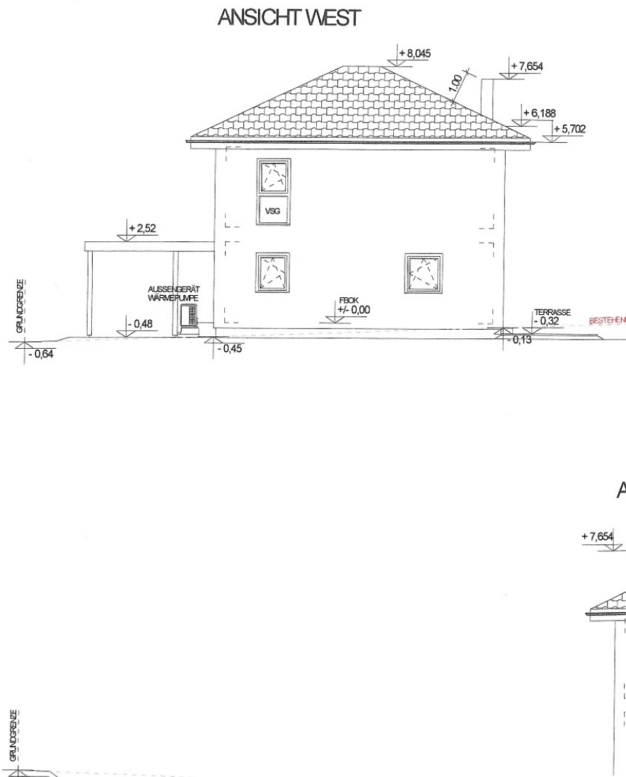
Neues 117m 2 Einfamilienwohnhaus in Viktring
