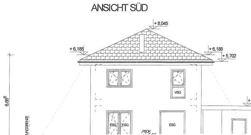
Neues 117m 2 Einfamilienwohnhaus in Viktring
