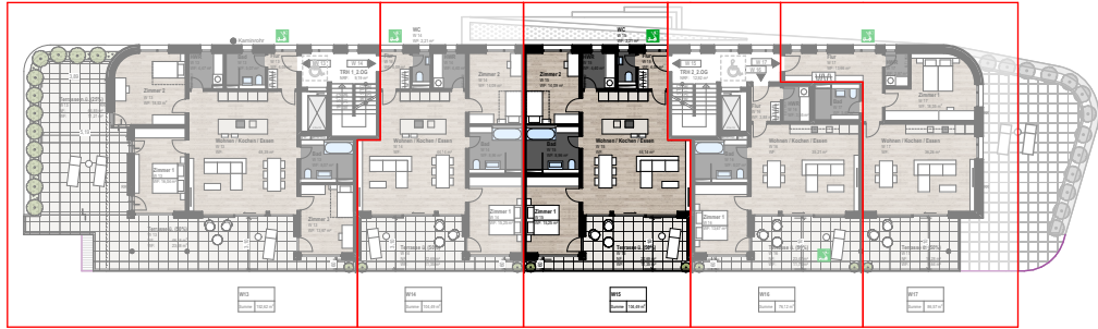
2.Obergeschoss M1:500
