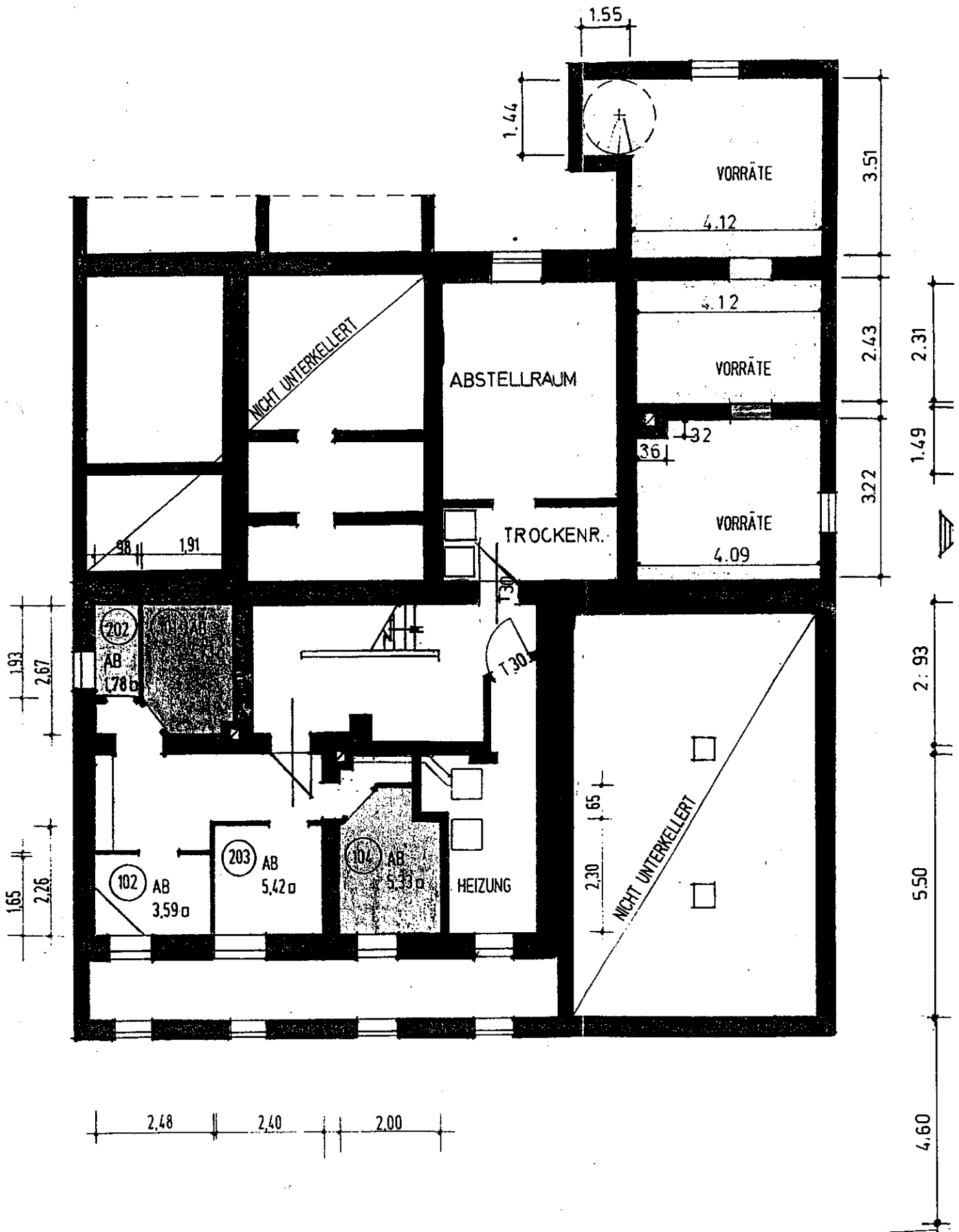
KELLERGESCHOSSGRUNDRISS M/1/100
