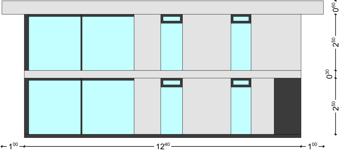
Ansicht Ost
