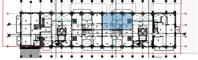
OBERGESCHOSS 2
