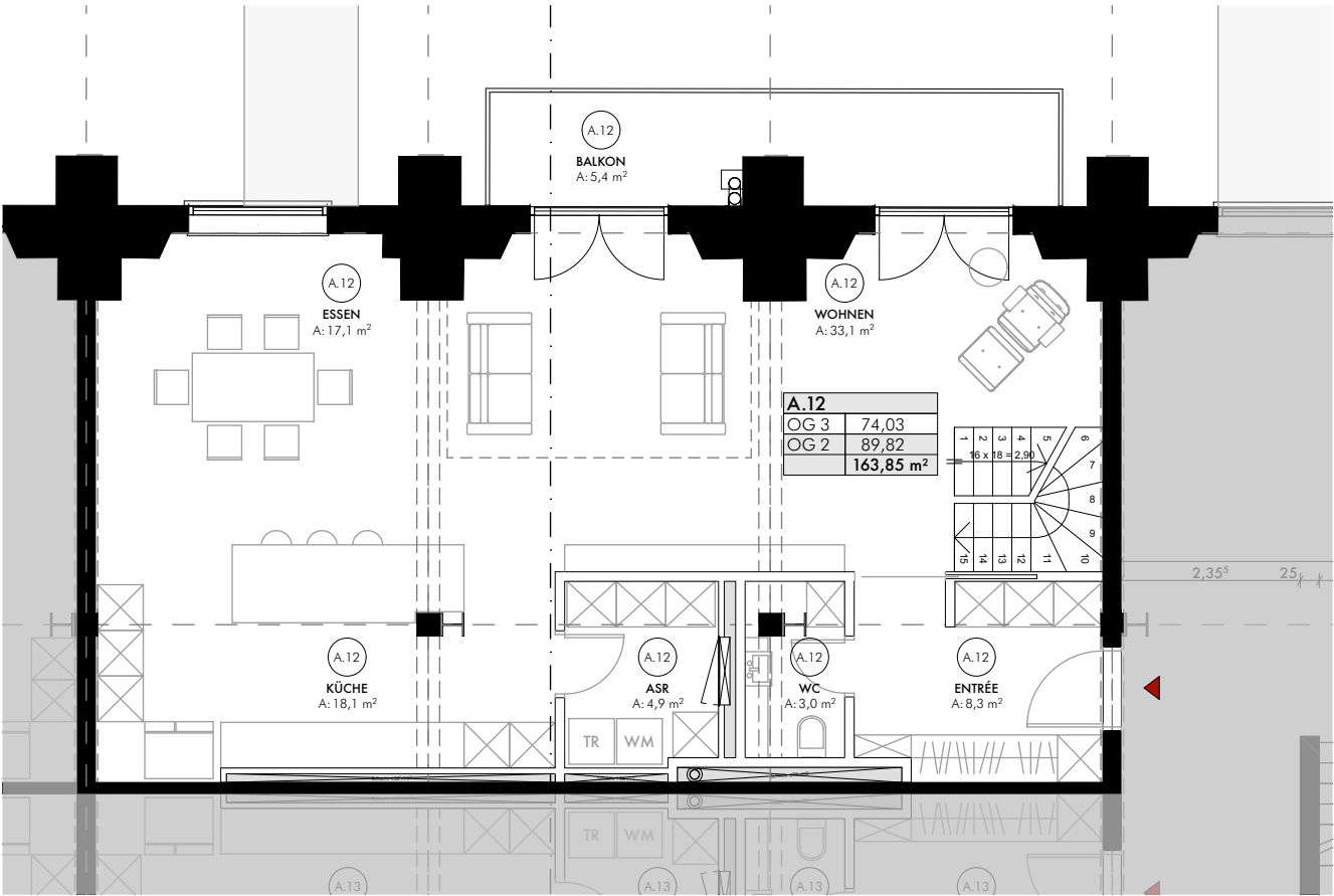
OBERGESCHOSS 2
