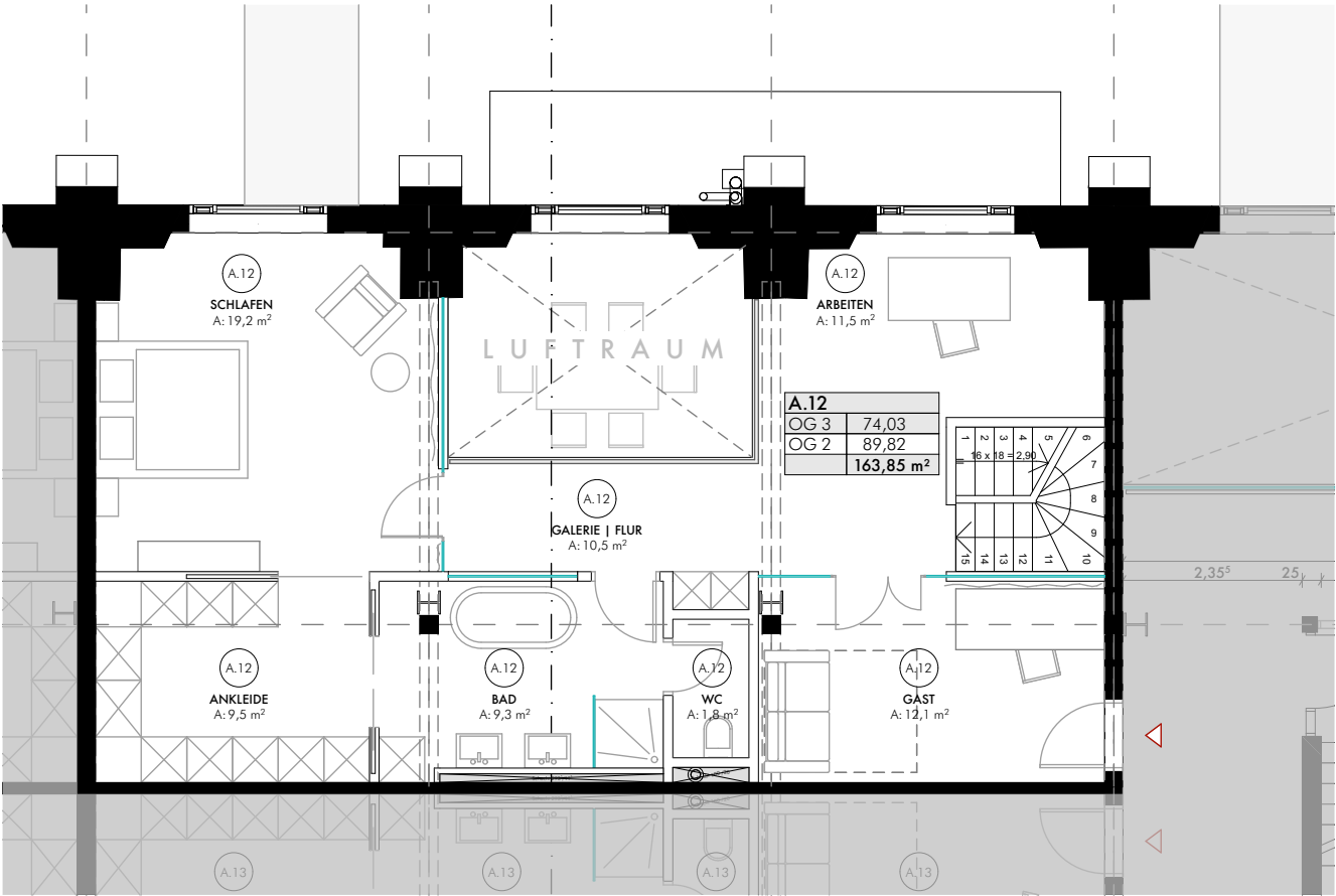
OBERGESCHOSS 3
