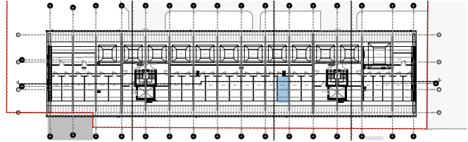
OBERGESCHOSS 5
