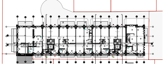
ERDGESCHOSS
