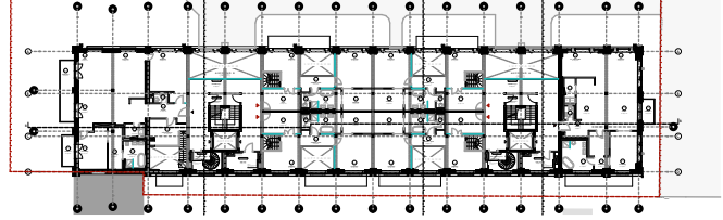
OBERGESCHOSS 4
