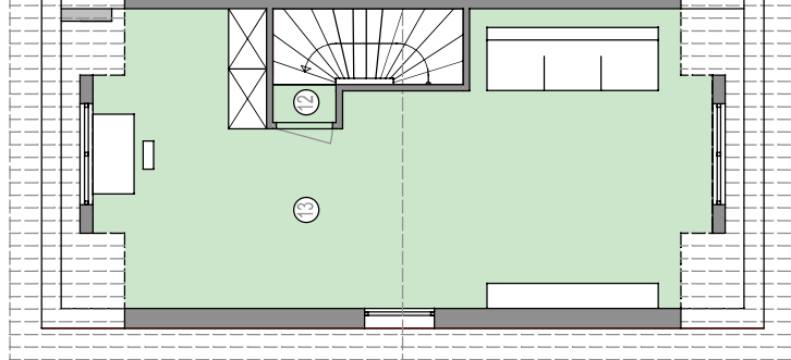
Grundriss Dachgeschoss
