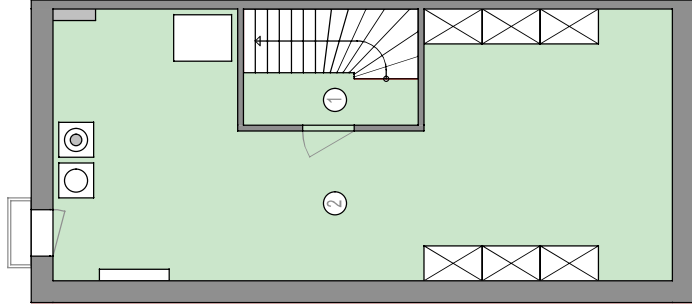
Grundriss Kellergeschoss
