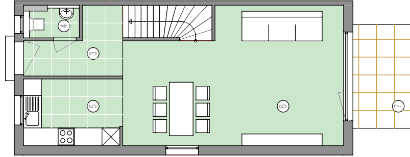
Grundriss Erdgeschoss
