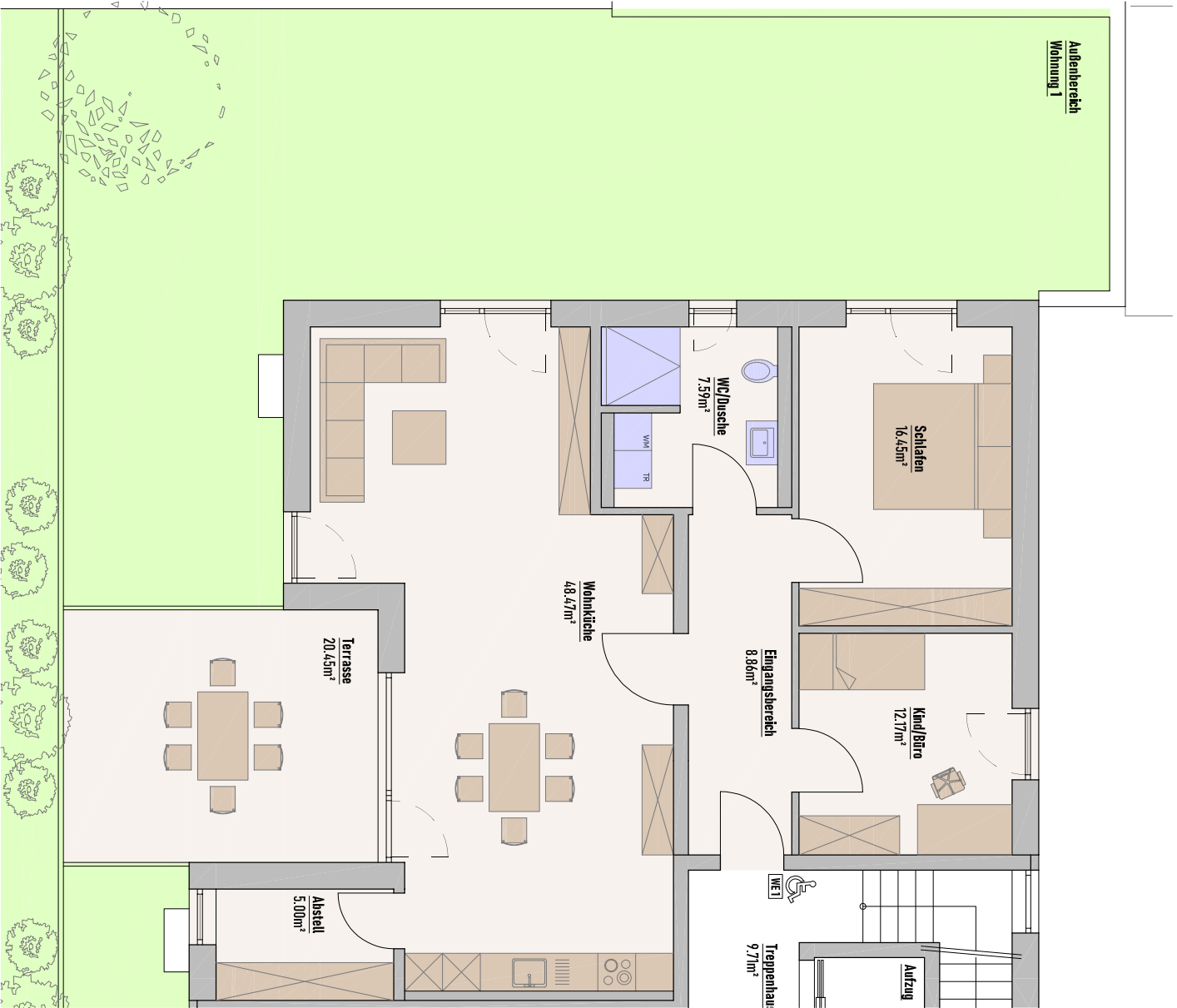
Erdgeschoss
