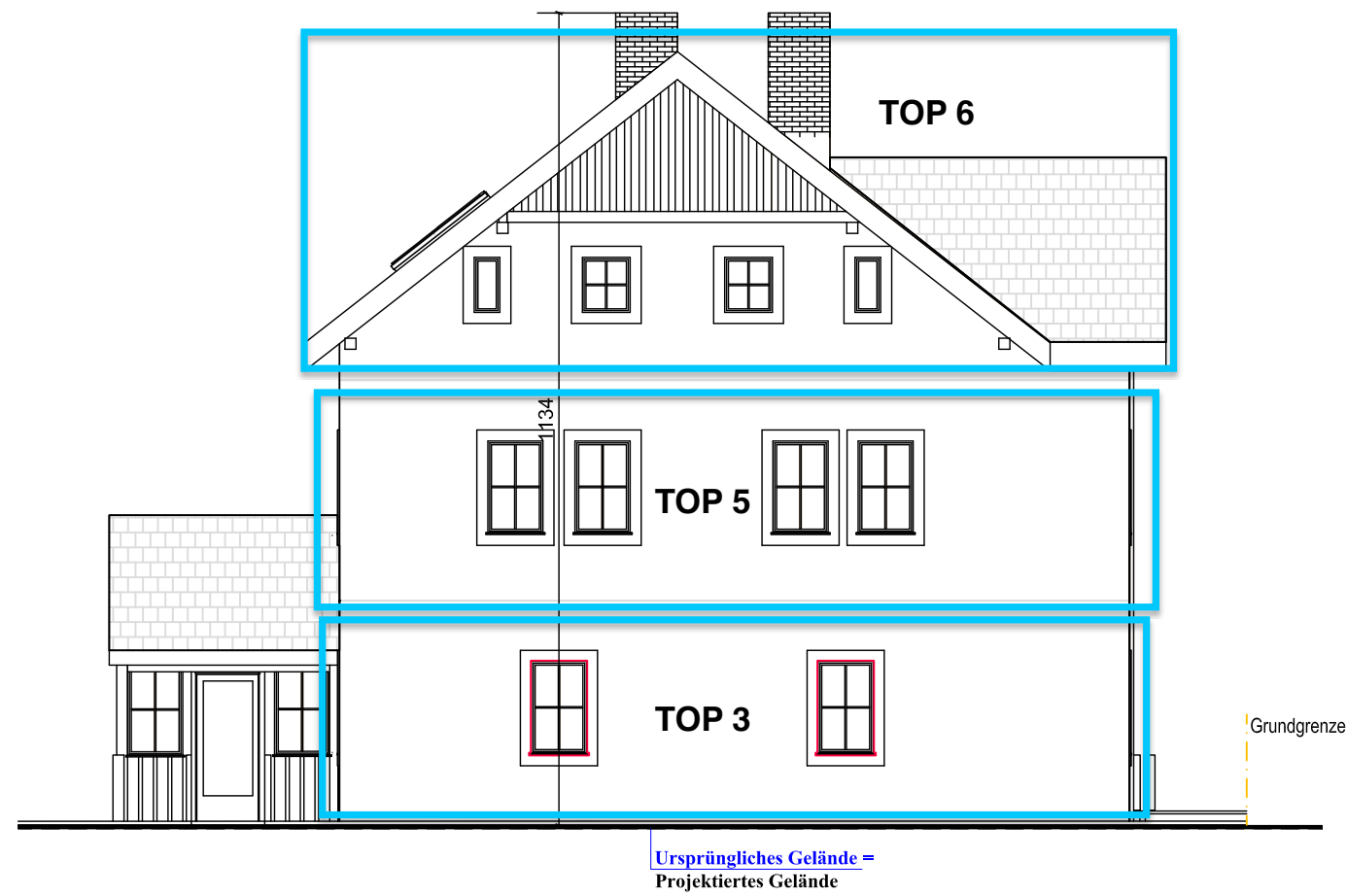
ANSICHT NORDEN
