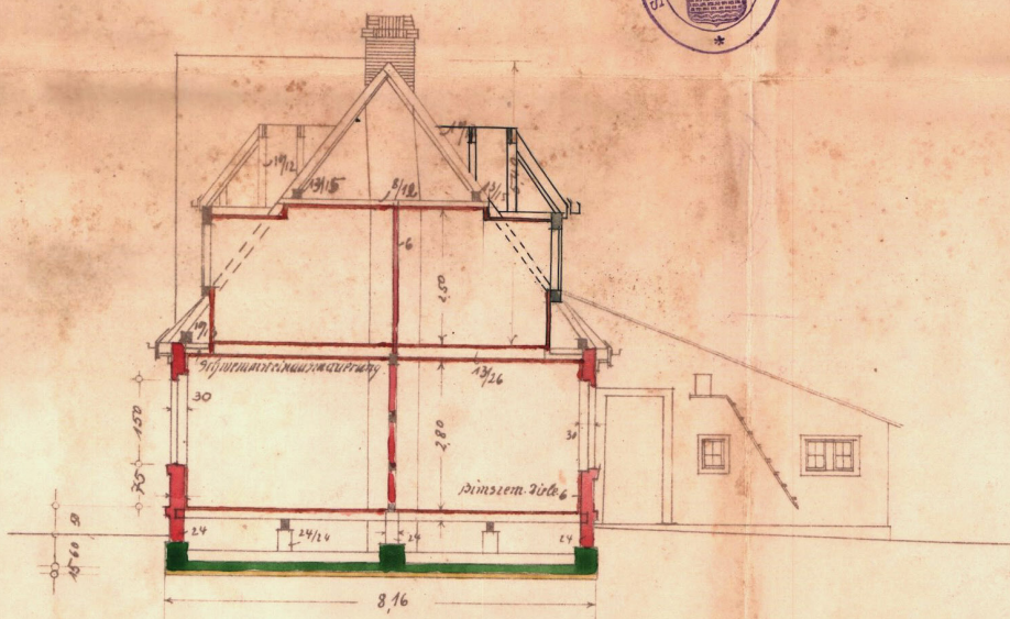
Querschnitt M: 1:100
