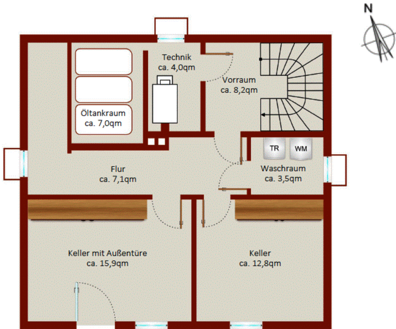
Grundriss KG
