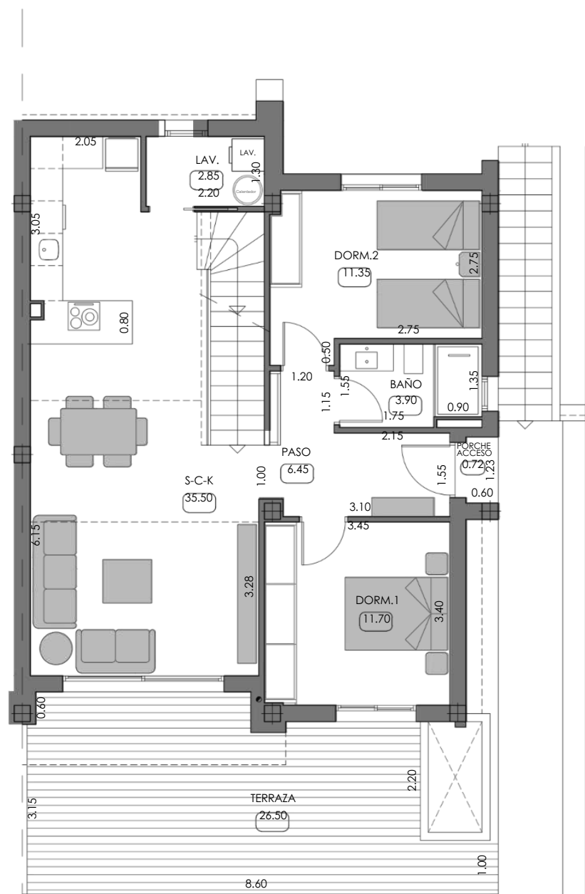
PLANTA BAJA
