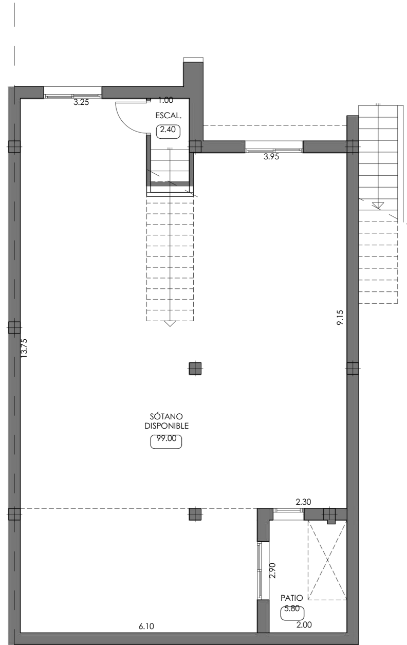
PLANTA SÓTANO
