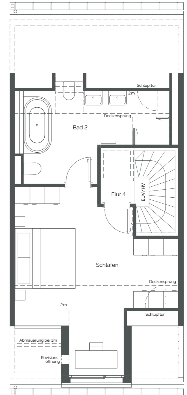
Dachgeschoss
