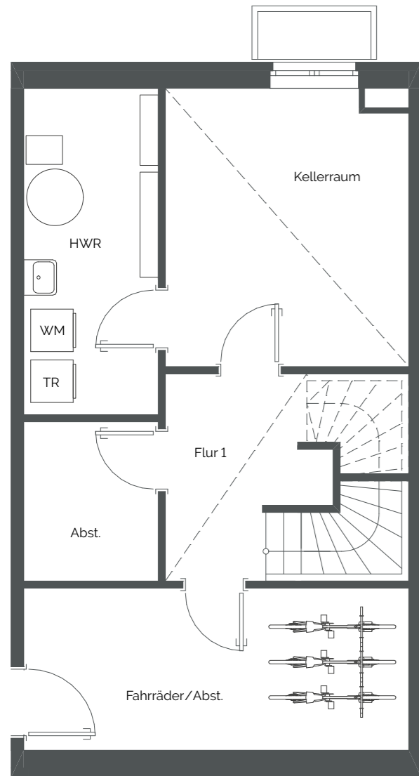
Kellergeschoss
