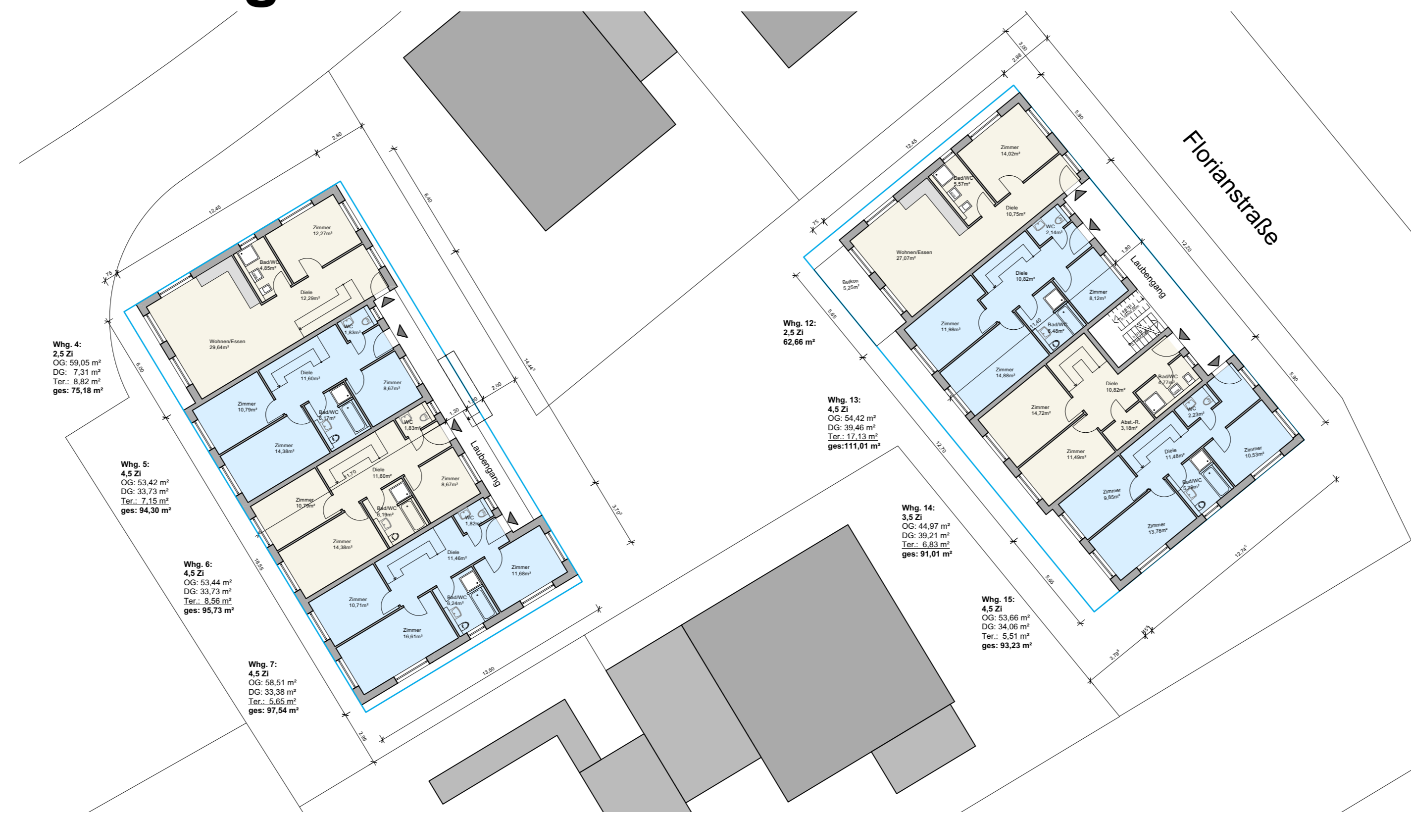
1. Obergeschoss
