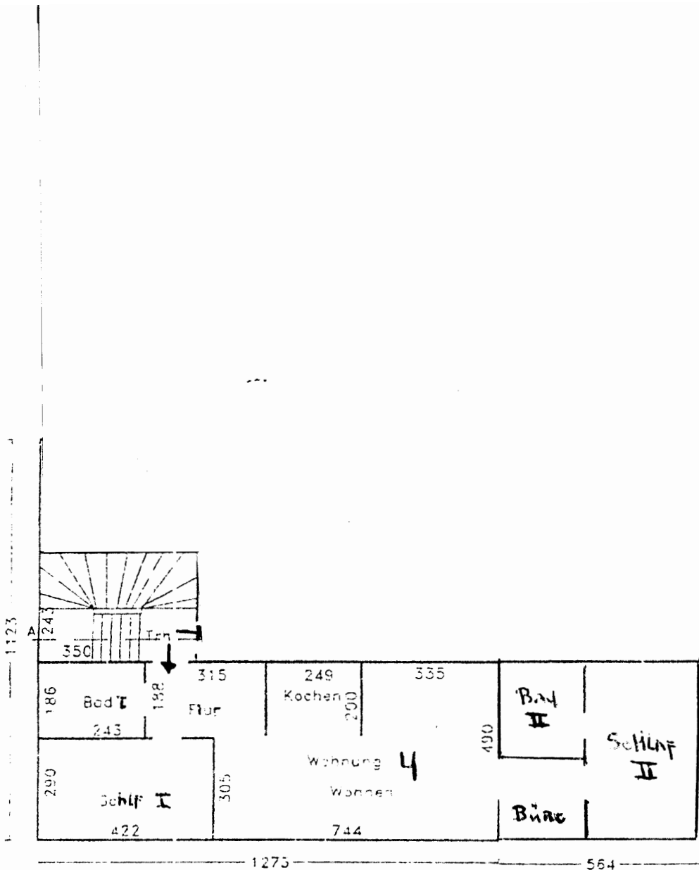
Grundriß II. Obergeschoß Wohn- und Geschäftshaus II OG.
