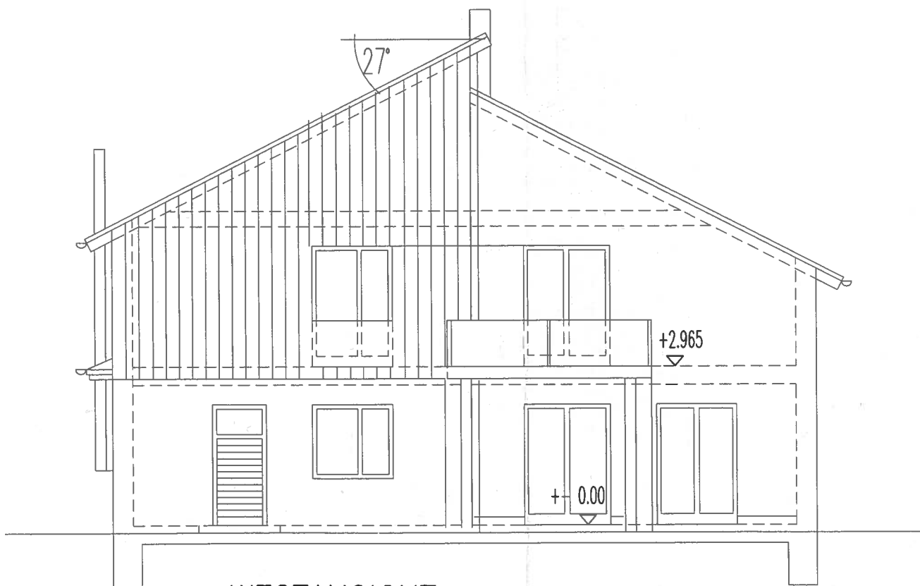
WESTANSICHT
