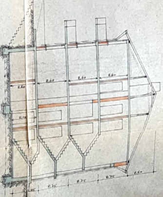
QUERSCHNITT
