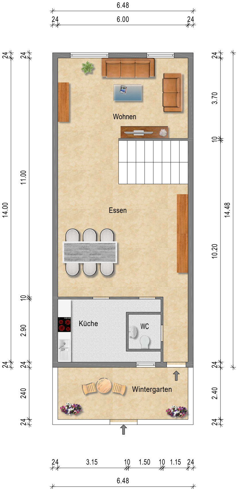
Erdgeschoss
