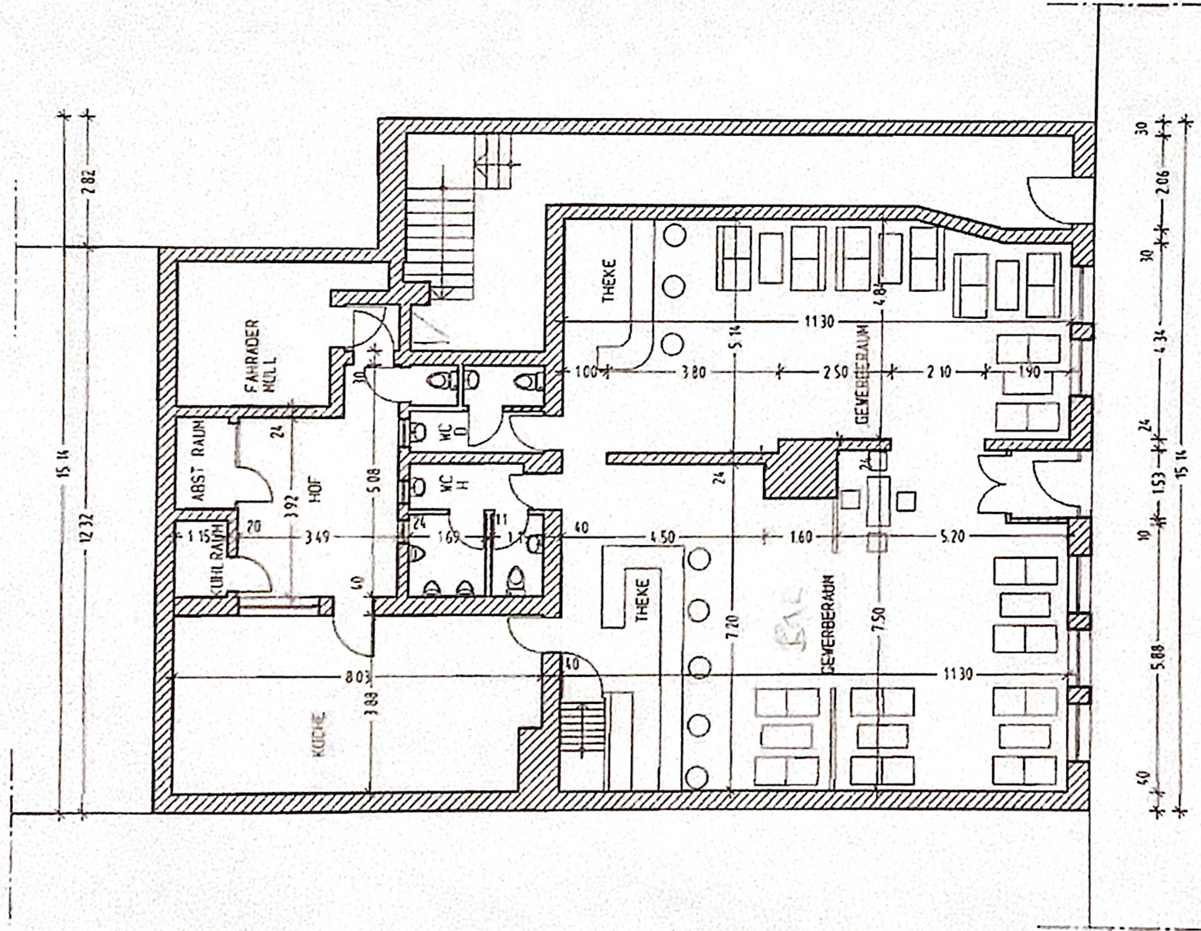
GRUNDRISS ERDGESCHOSS S1,15
