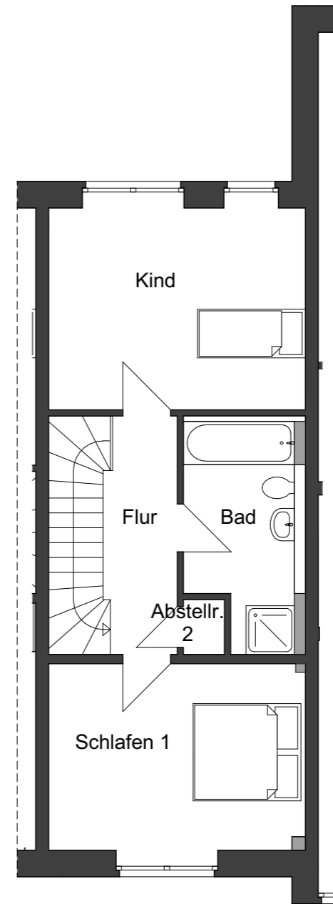
Grundriss 1.OG
