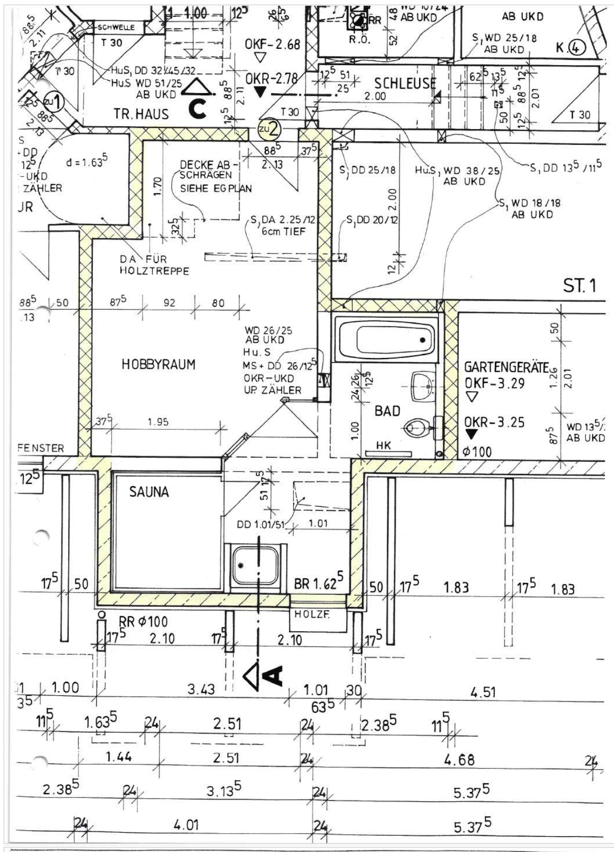
Grundriss UG
