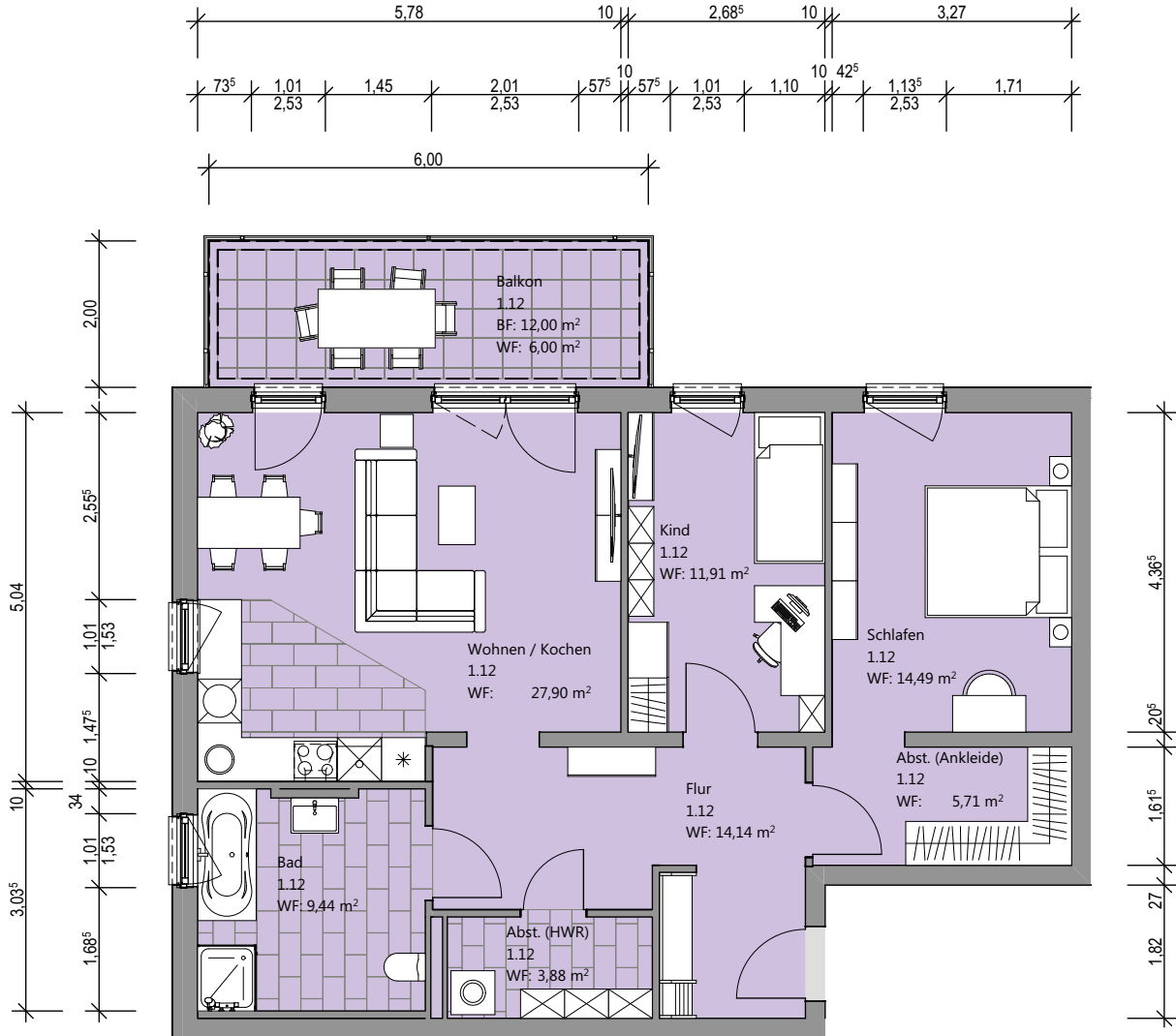
Wohnung 1.12
