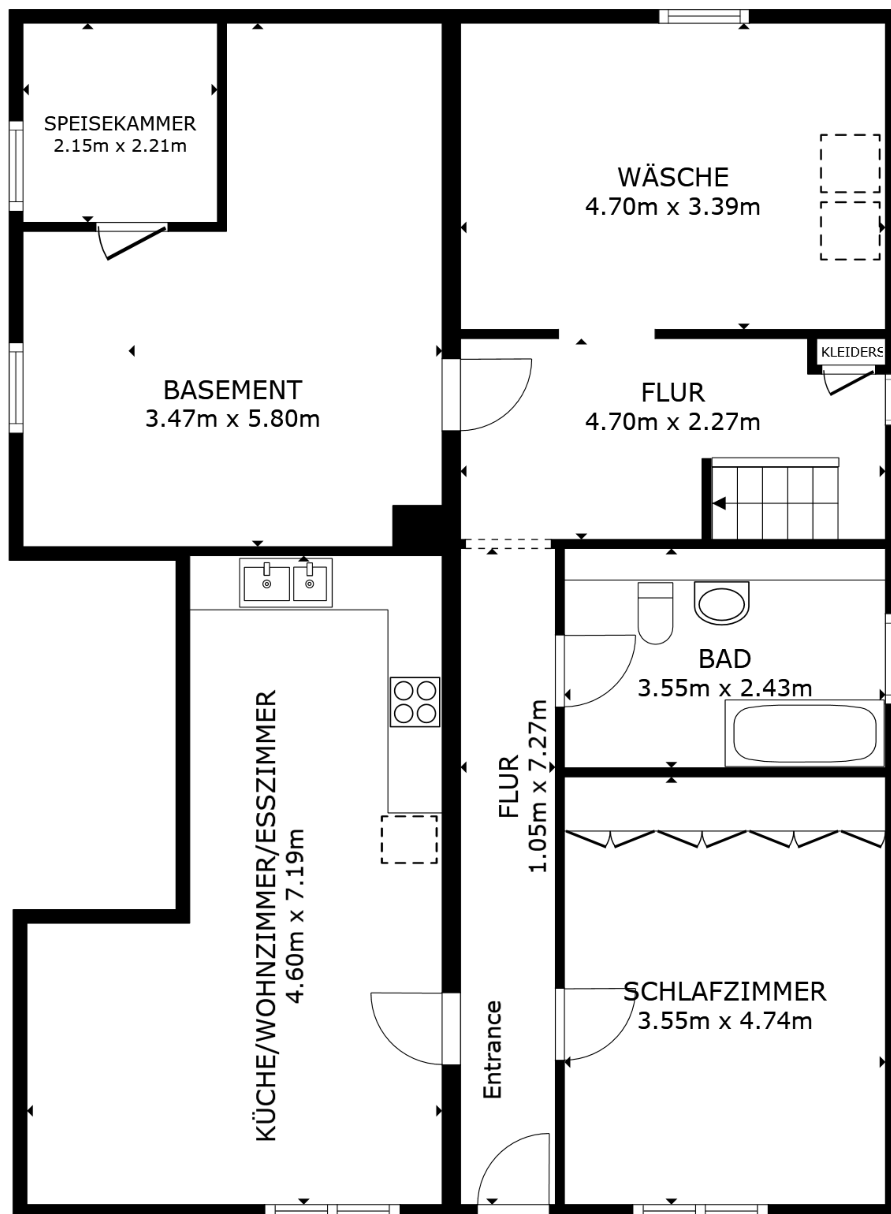
STOCKWERK 1
