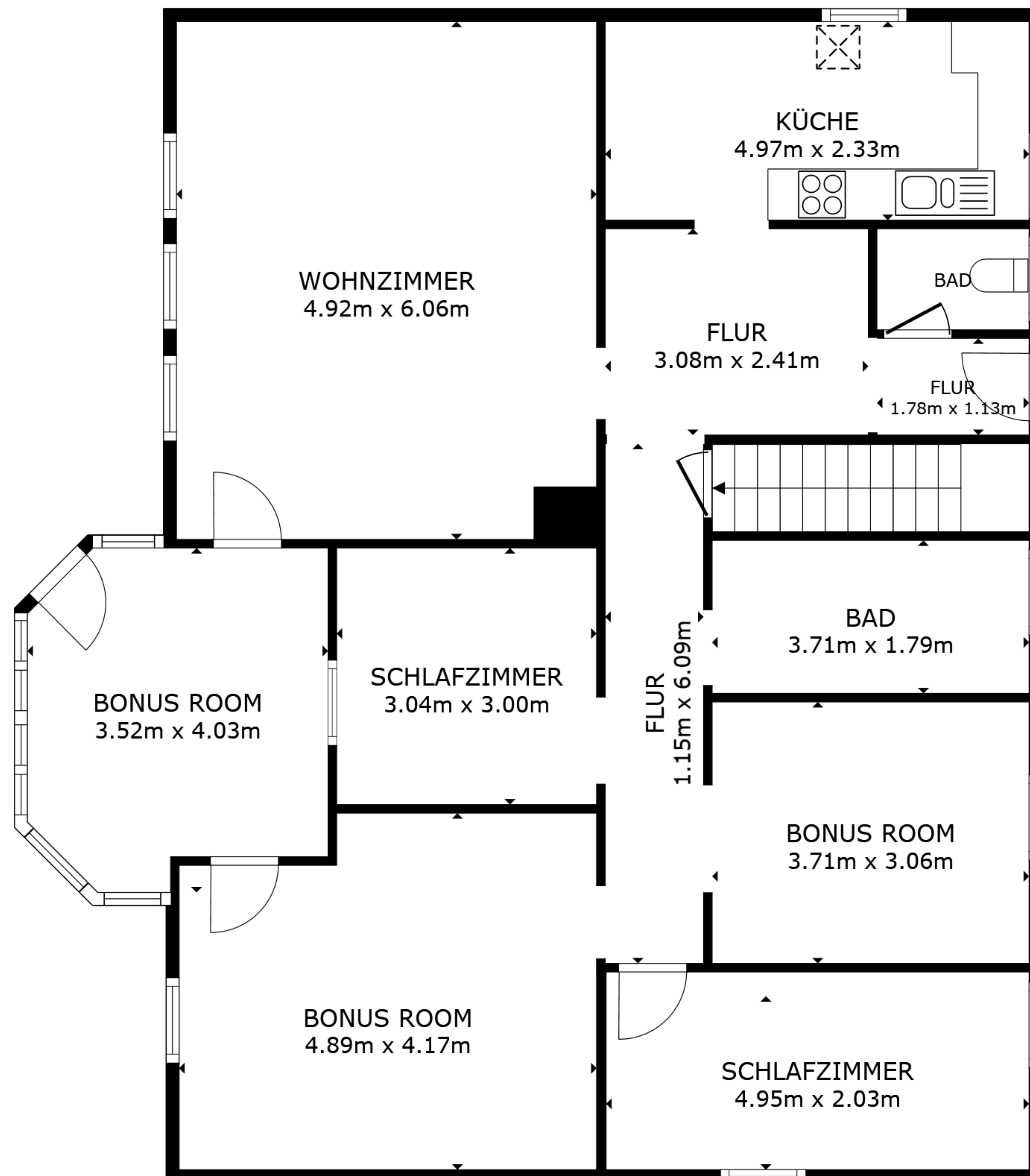
STOCKWERK 2
