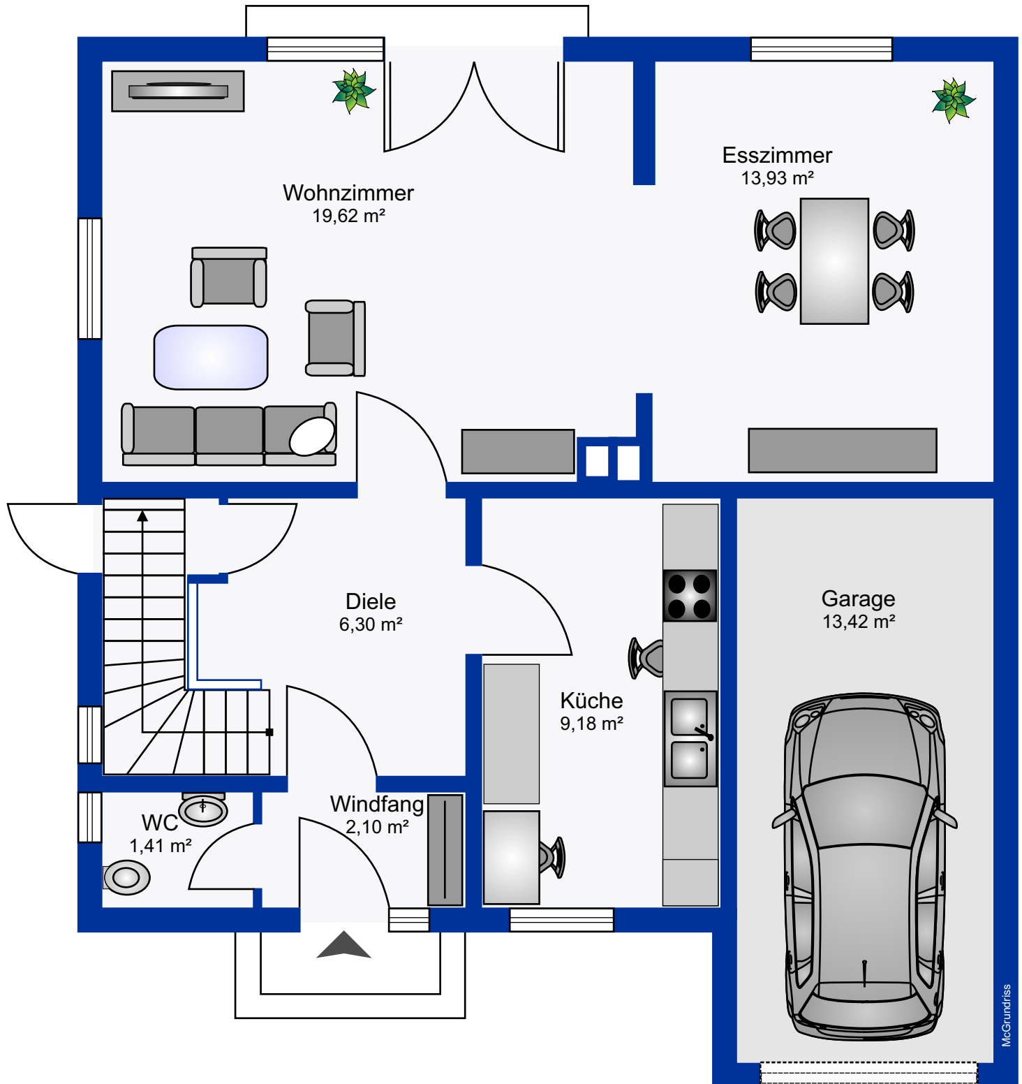
Erdgeschoss
