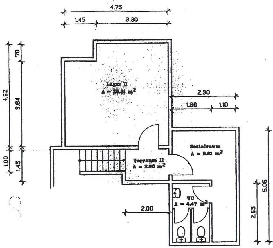
Grundriss Ebene +1.66 m
