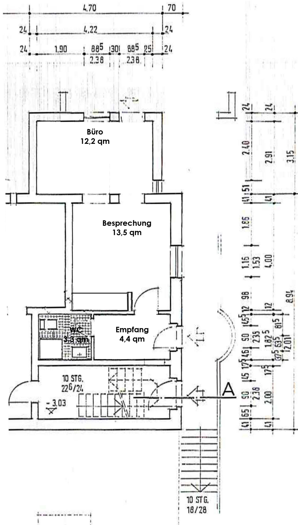
Grundriss Büro
