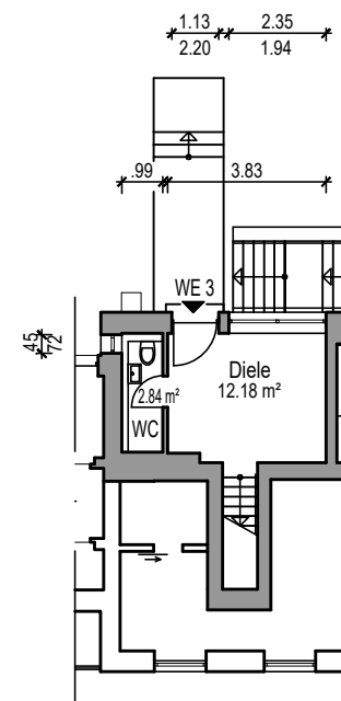
Grundriss WE3 OG1
