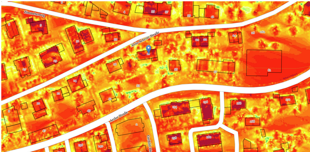
Sonnenscheindauer 21. Jun
