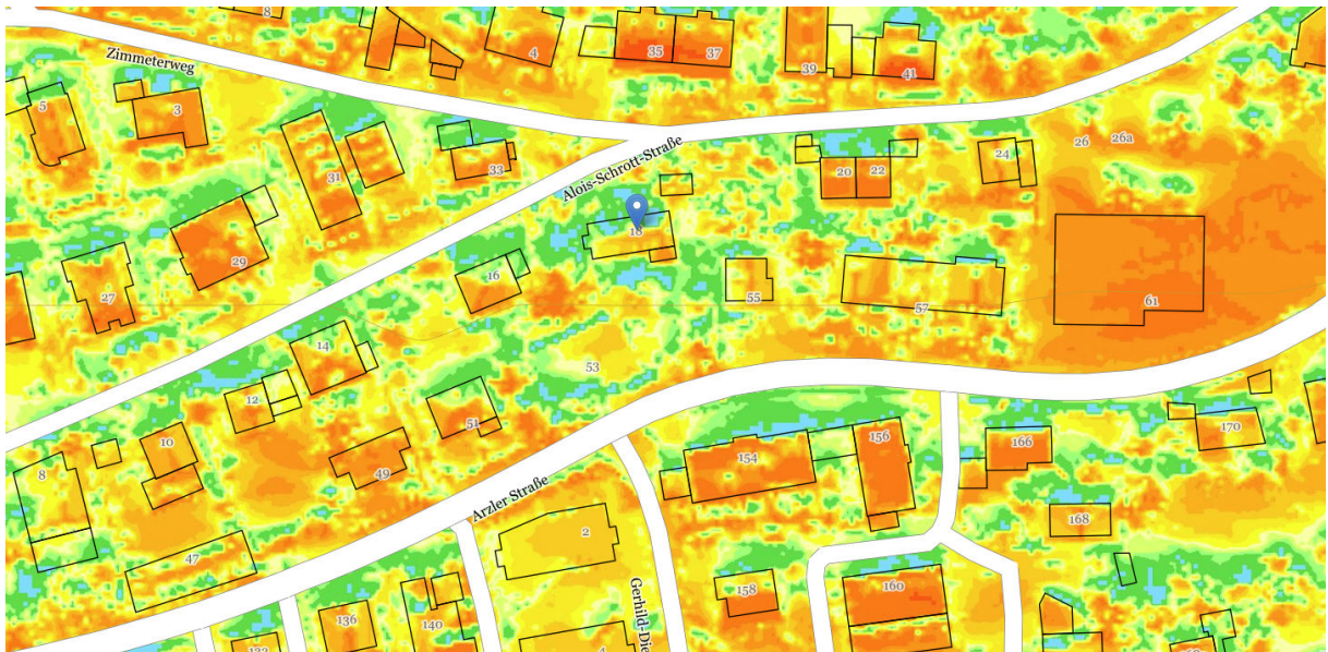
Sonnenscheindauer 21. Feb
