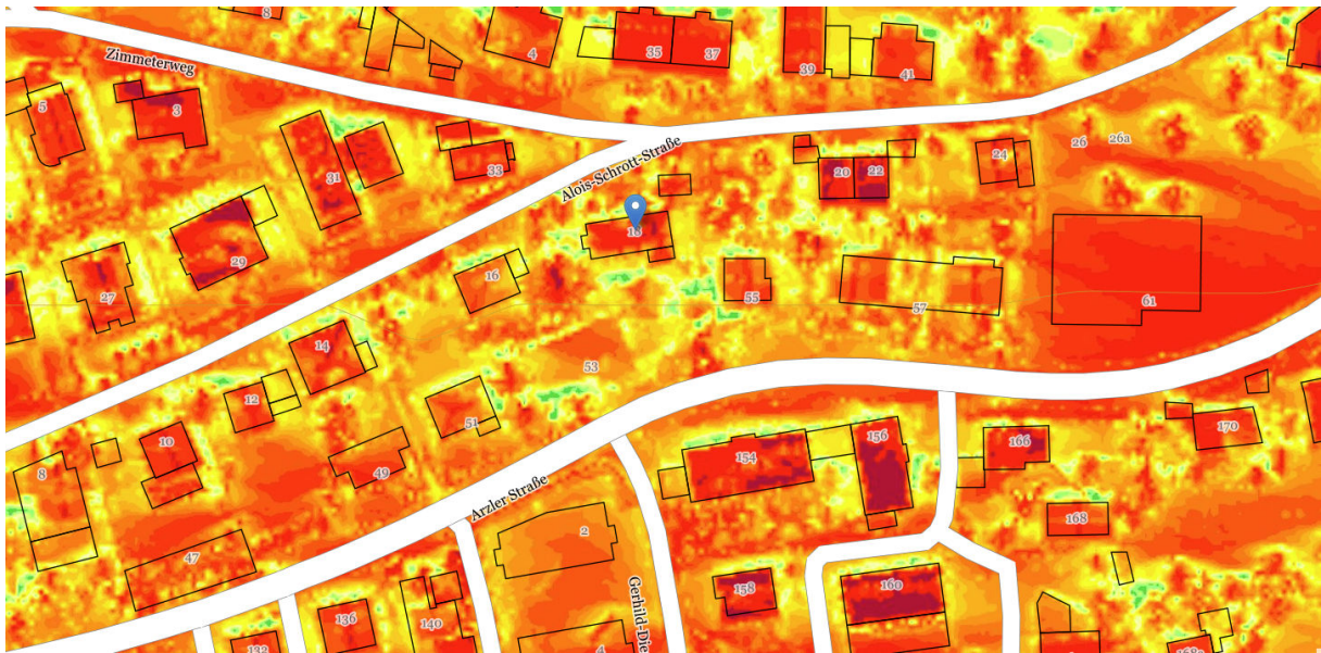
Sonnenscheindauer 21. Mai
