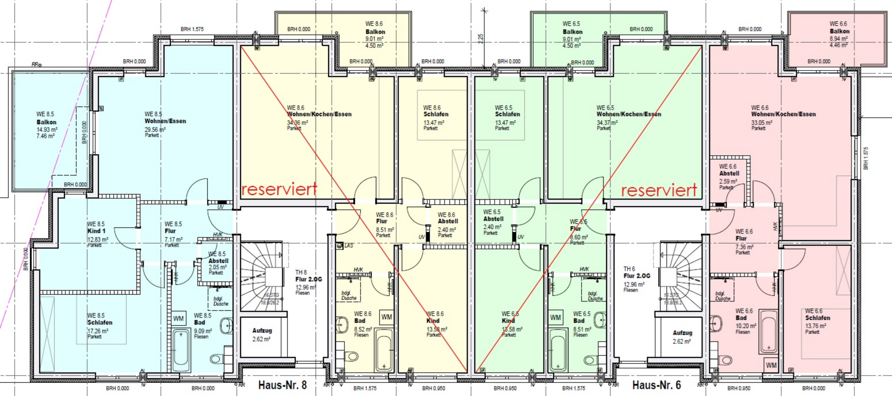
Grundriss 2.Obergeschoss Haus 6 und 8
