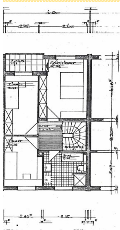
Dachgeschoss
