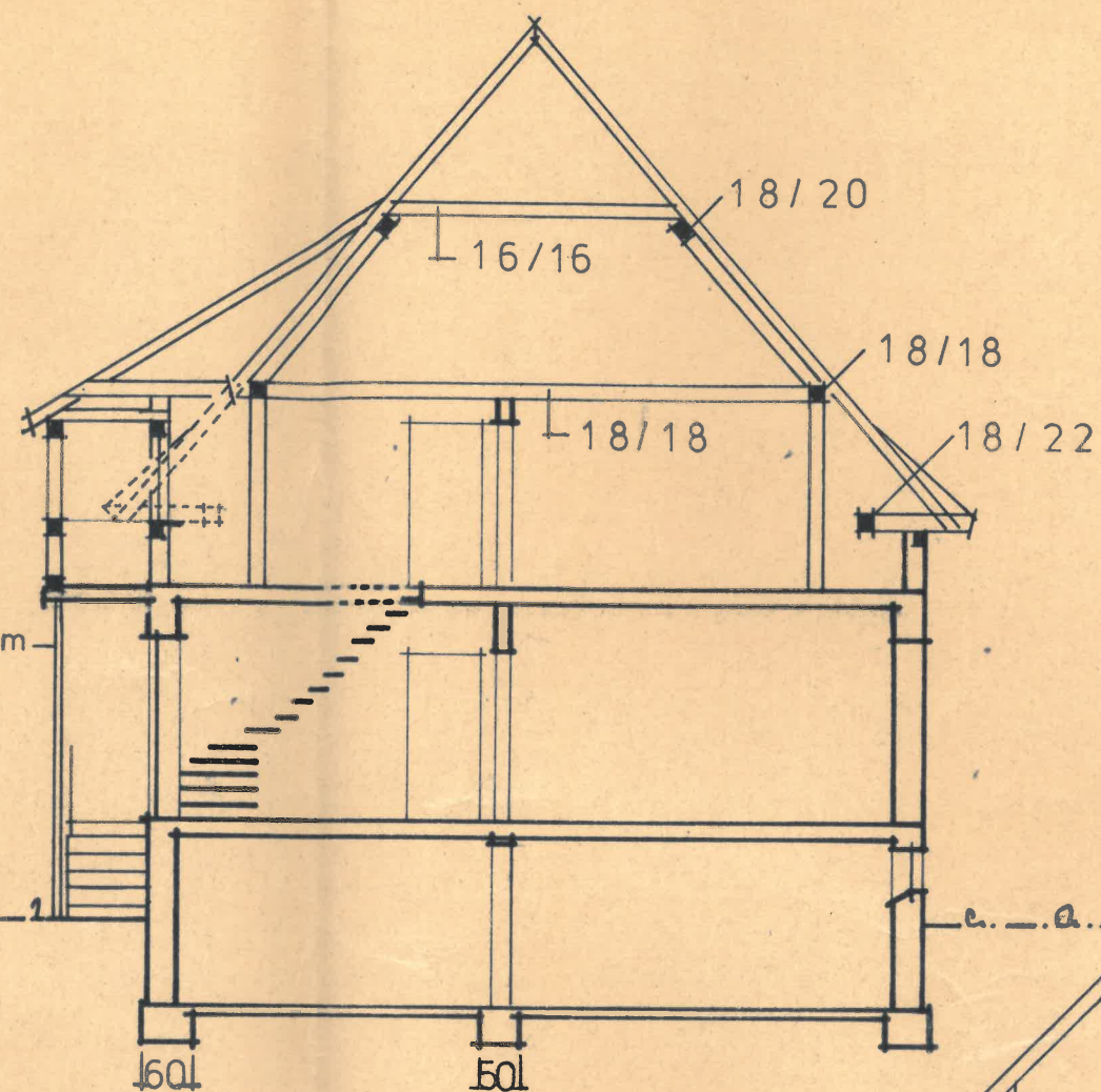
SCHNITT A-3
