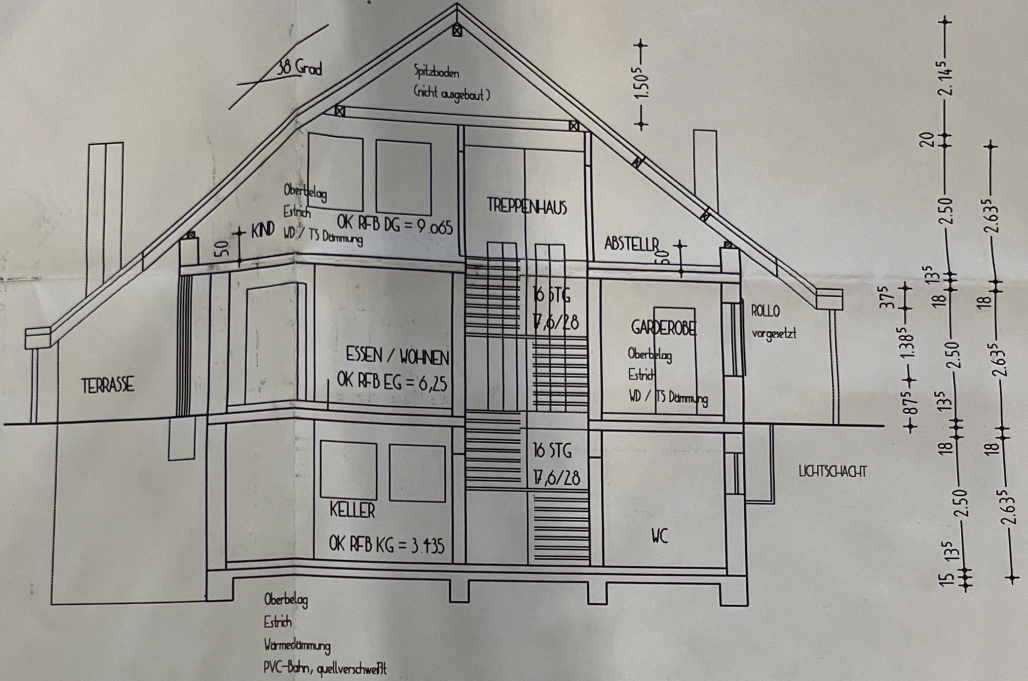
SCHNITT 1-1 M.1 : 100
