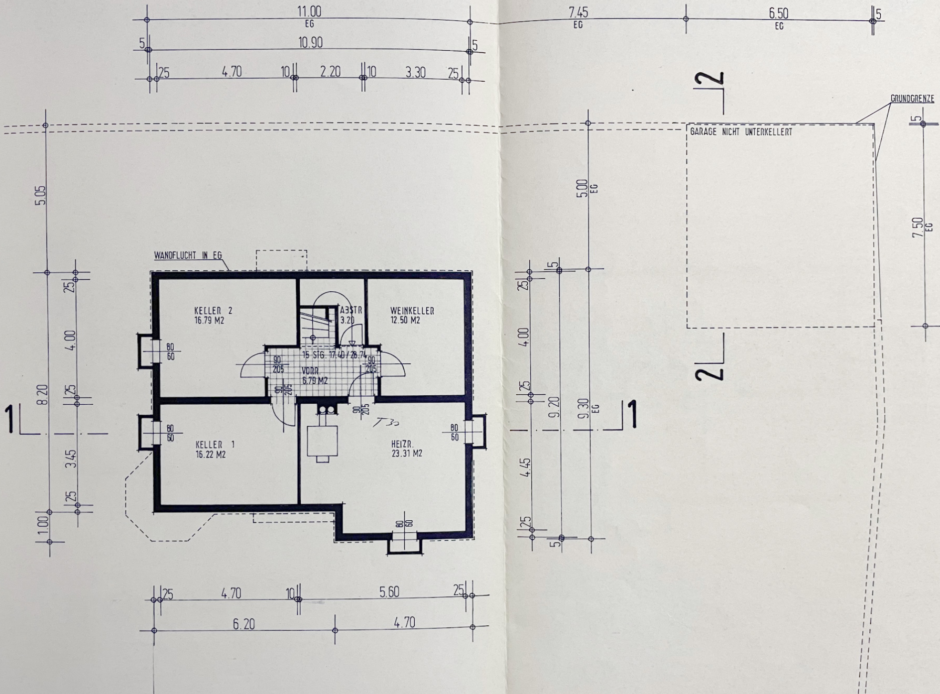
GRUNDRISS UNTERGESCHOSS
