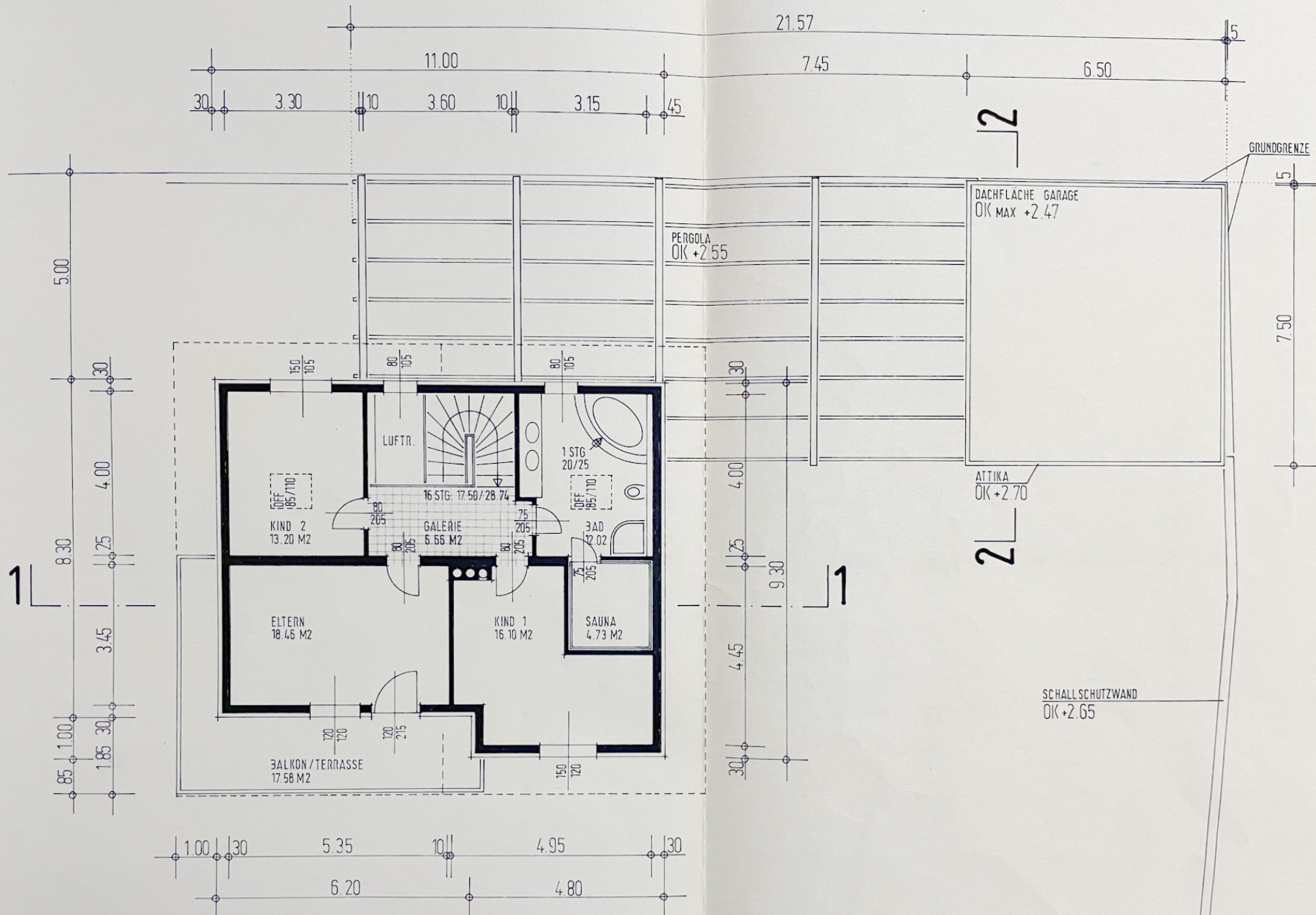
GRUNDRISS DACHGESCHOSS
