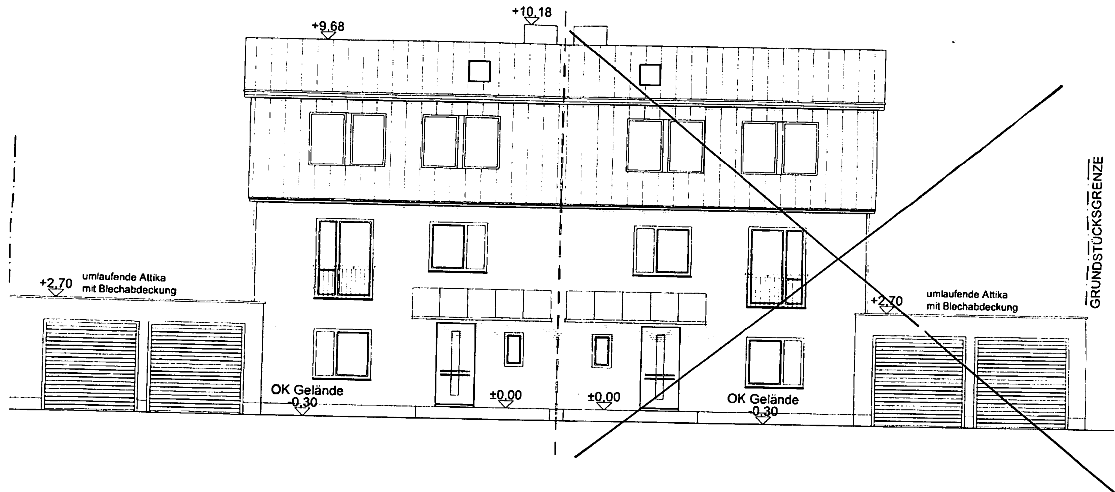
ANSICHT VON NORD-OSTEN HAUS 1 und 2
