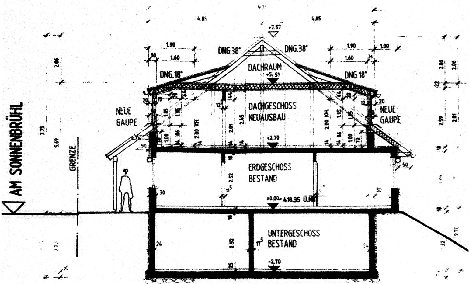
QUERSCHNITT ZUM AUSBAU DES DACHGESCHOSSES UND NEUAUFBAU DER DACHGAUPEN
