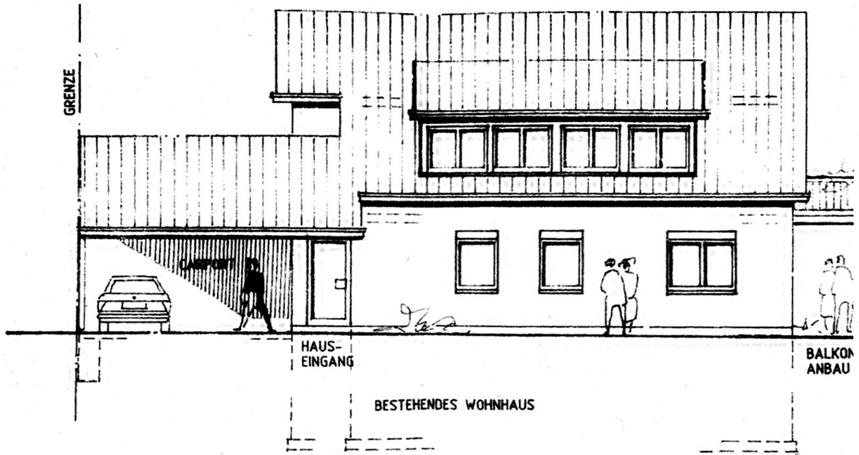
NORD-U. STRASSENANSICHT
