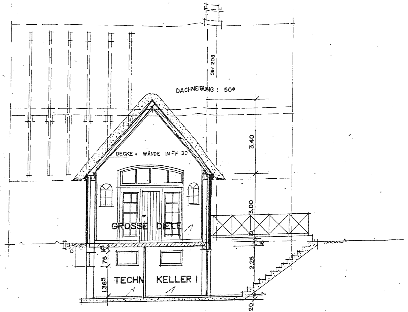
SCHNITT B...B
