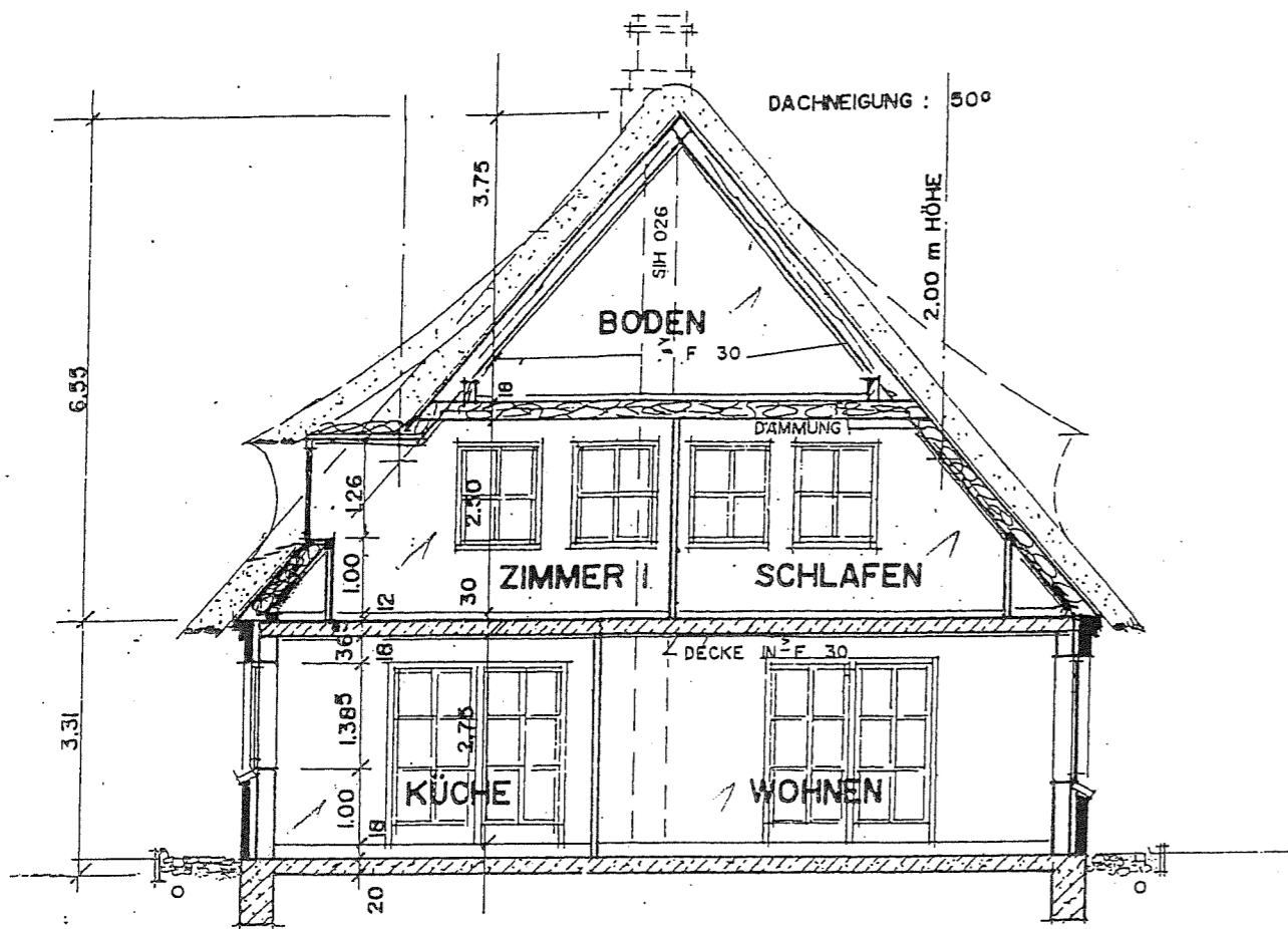
SCHNITT A...A
