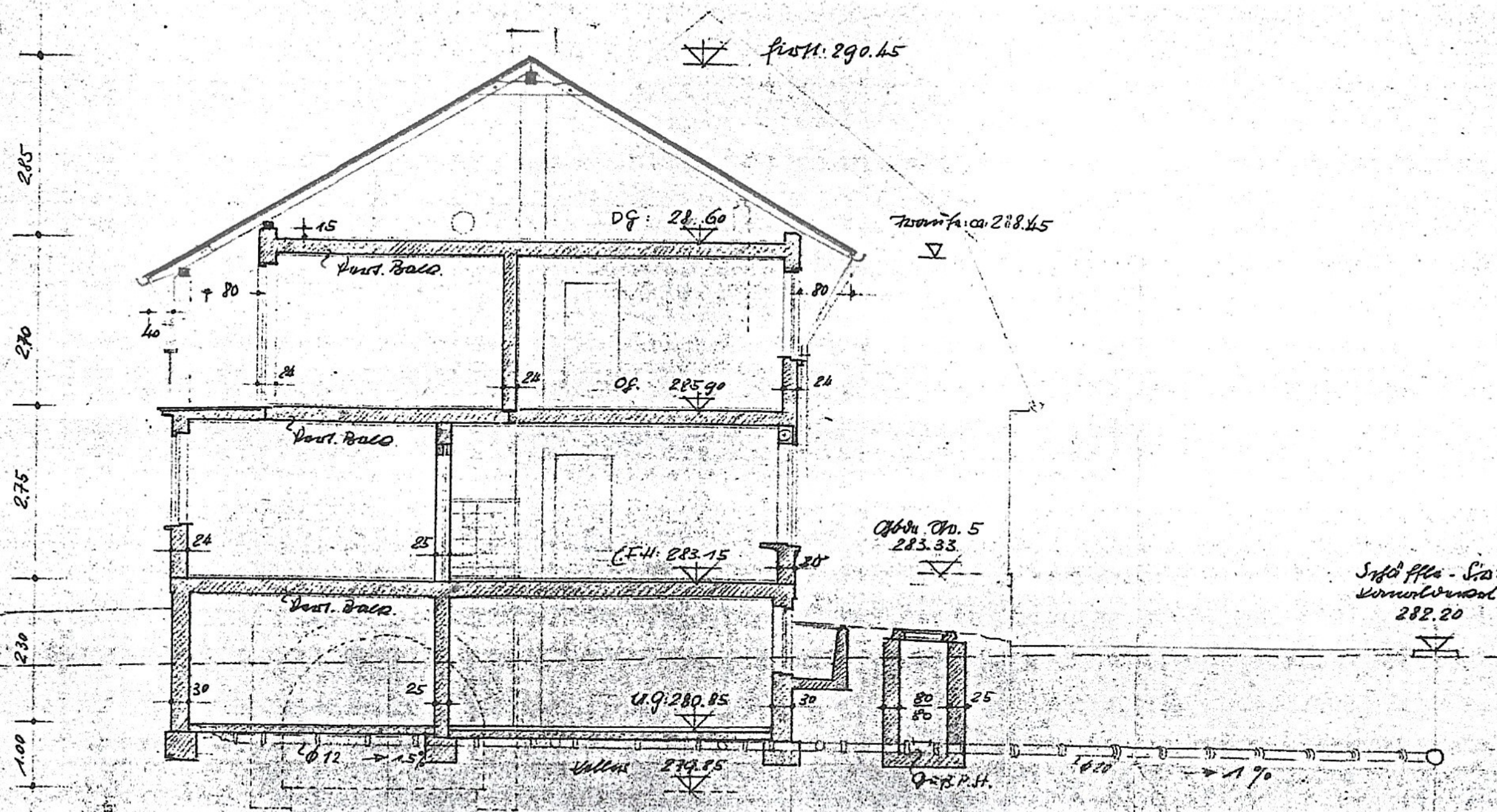
SCHNITT WOHNHAUS
