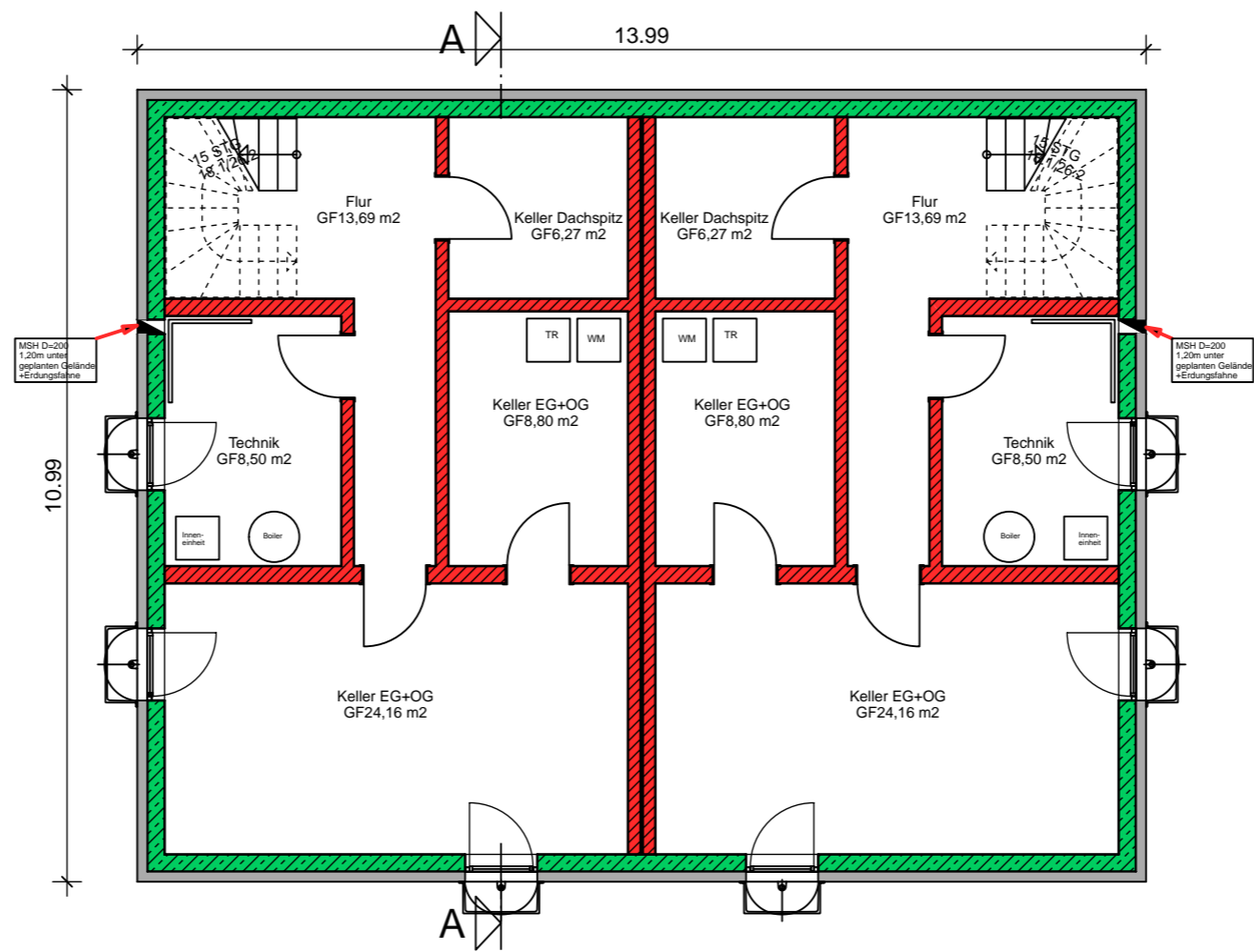
Kellergeschoss
